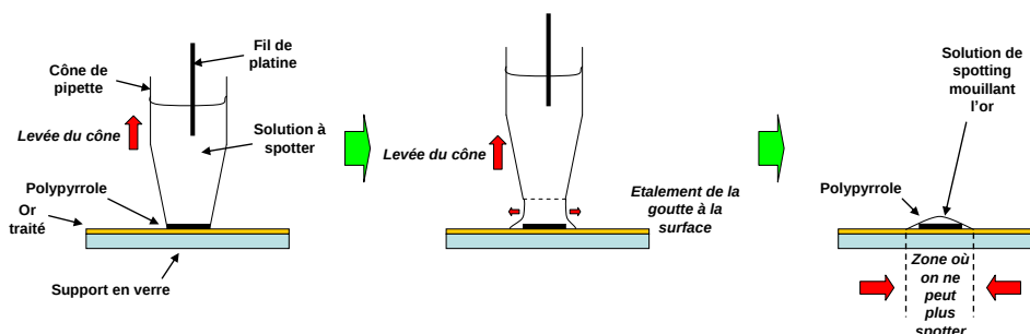
Figure 64 : Représentation schématique du principe de mouillage du milieu à polymériser sur la surface dorée ; cas d'une surface traitée par alcane-thiols
