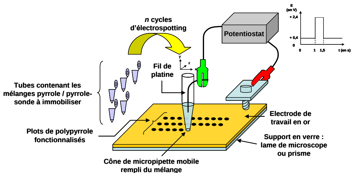
Figure 4 : Représentation schématique du robot Polypotter conçu pour la fabrication de biopuces par électrospotting ; les commandes de déplacement de la cellule électrochimique sont pilotées par logiciel développé au laboratoire
