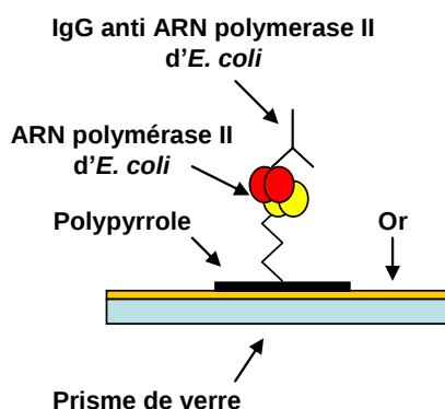
Figure 74 : Principe de la caractérisation de l'ARN polymérase II d' E. coli suivant le modèle antigène / anticorps
