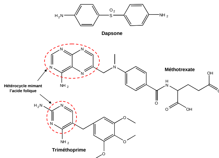
Figure 12 : Structure d'une sulfone, la dapsone (Disulfone ® ), et de deux inhibiteurs de la dihydrofolate déshydrogénase, le triméthoprim (Bactrim ® ) et le méthotrexate (Methotrexate ® )
