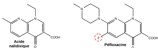
Figure 14 : Structure d'une quinolone, l'acide nalidixique (Negram ® ), et d'une fluoroquinolone, la péfloxacin (Péflacine ® )
