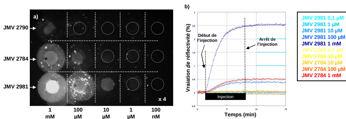
Figure 49 : a) Image de fluorescence d'une puce biotine / FITC r2v2l2e2e par la SAPE – b) Cin2tiques obtenues apr2s injection de 100 nM d'anticorps monoclonal anti-biotine sur une puce biotine
