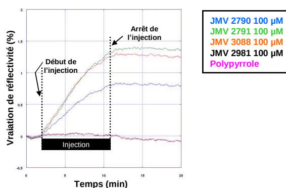
Figure 50 : Cin2tiques obtenues apr2s injection de 100 nM d'anticorps monoclonal anti-FITC sur une puce FITC/biotine
