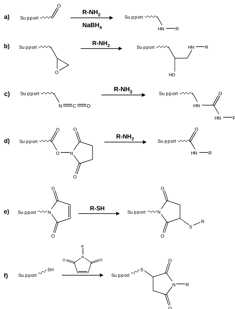
Figure 23 : Différentes chimies de greffage covalentes « non régio-sélectives » développées pour les peptides et les protéines – a) par aldéhyde [59] – b) par GTPS [60] – c) par isocyanate [61] – d) N -hydroxysuccinimide [61] – e) par maléimide [62] – f) par thiol
