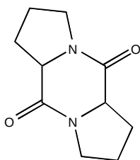
Figure 34 : Cyclodipeptide ayant une activité antibiotique selon Huberman et al [118]
