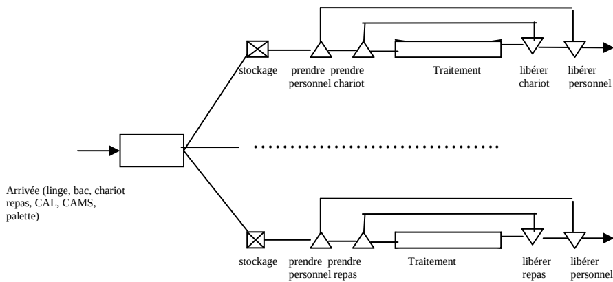
Figure 3.2.3 : Modèle de files d'attente
