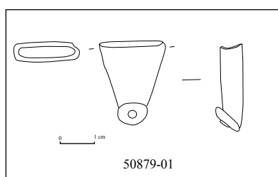
Fig. 118 : Autre type de bouterolle découverte à Salins
