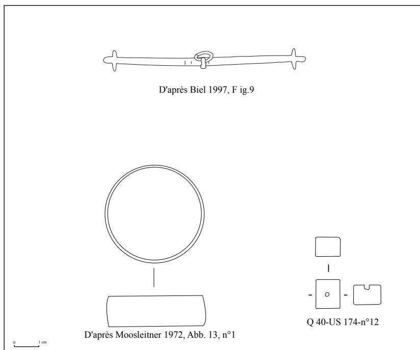
Fig. 68 : Éléments liés aux instruments de mesure issus des sites de Hochdorf, Bourguignon-les-Morey et du Hellbrunnenberg
