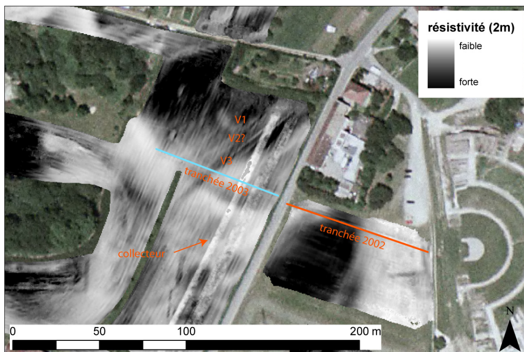
Figure 182. Mandeuve (Doubs). Carte de la résistivité électrique du sol (dispositif ARP à 2m). Localisation des tranchées géoarchéologiques 2002-2003, du collecteur antique et des voies (V1, V2, V3) menant au sanctuaire (C. Laplaige, 2011. Source Geocarta/PCR Mandeuve)
