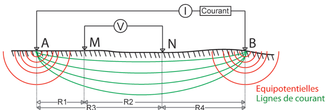
Figure 26. Schéma figurant le principe de la prospection électrique (C. Laplaige, 2011)
