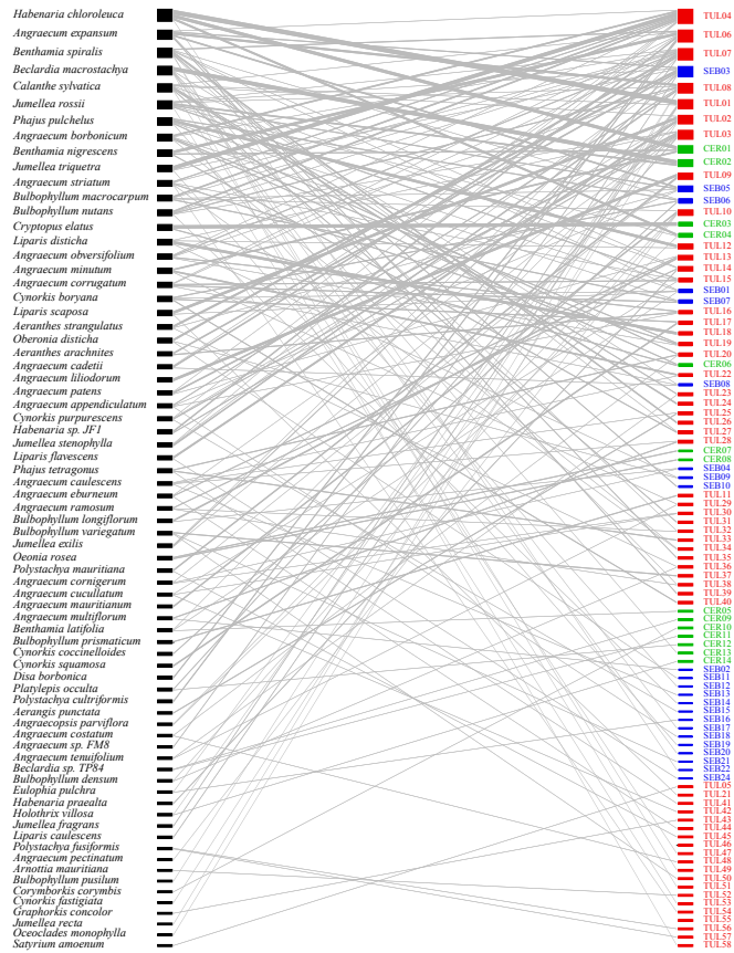
FIGURE 9.1 – Architecture emboîtée ( nestedness ) du réseau mycorrhizien formé dans les communautés d'orchidées autotrophes de La Réunion ( T=4.46 , P<0.001 ). Rouge : Tulasnellaceae ; bleu : Sebaciniales ; vert : Ceratobasidiaceae. Les partenaires sont ordonnés des plus généralistes (haut) au plus spécialistes (bas) des deux côtés du réseau.
