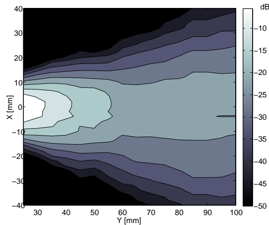
FIGURE 4.17 – Distribution de l'énergie rétrodiffusée par une bille avec l'élément numéro 64 dans le plan xOy . La région la plus claire correspond à une amplitude supérieure à -4.5 dB.
