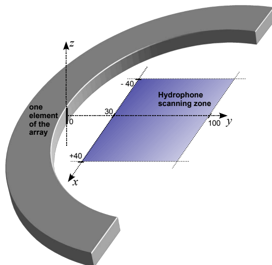
FIGURE 4.10 – Orientation du trièdre xyz par rapport à l’antenne semi-circulaire. Le plan d’inspection ( xOy ) est représenté.
