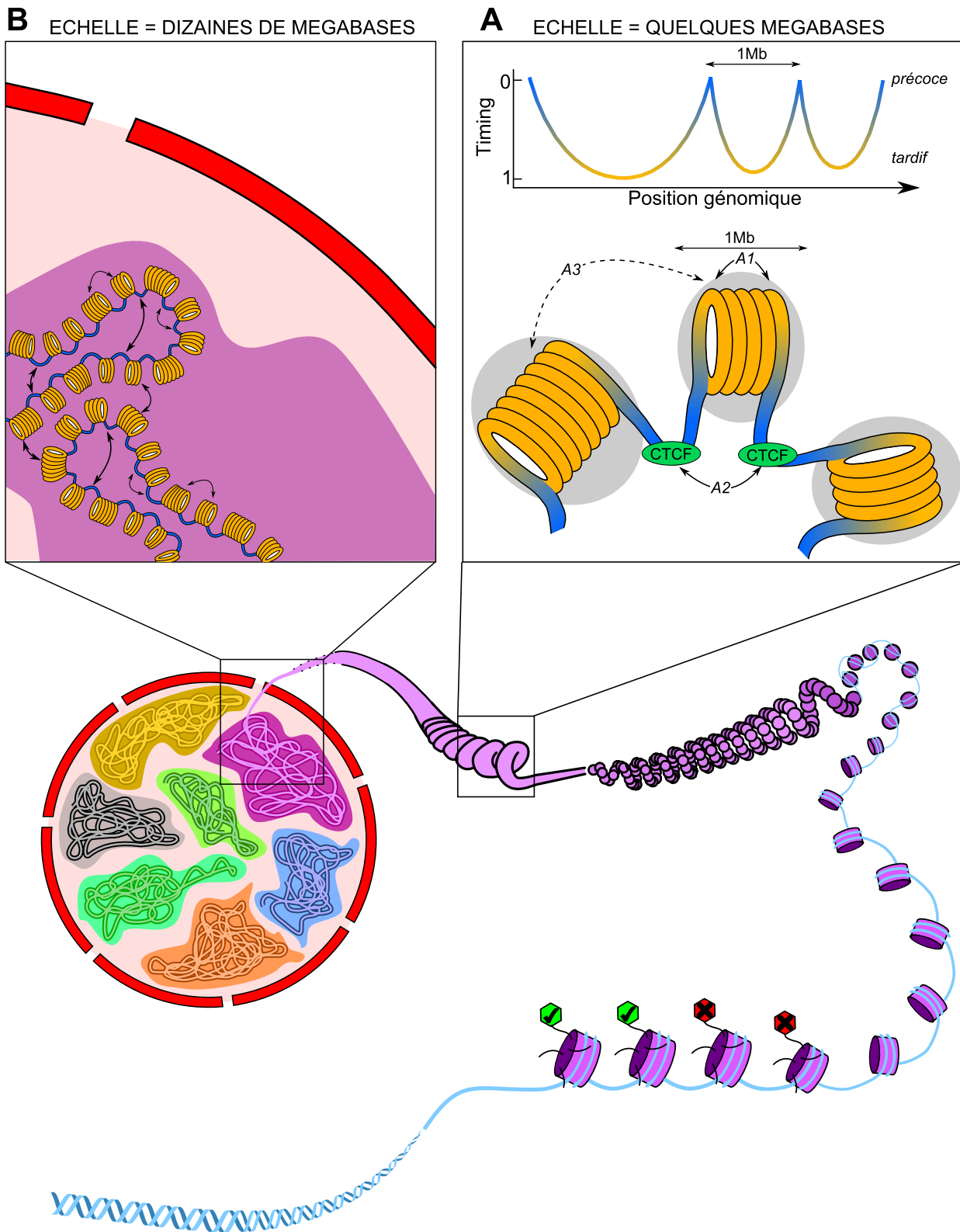
FIGURE 55 – Organisation topologique de la chromatine en suivant le timing de ré- plication. Ce schéma reprend celui de la figure 9. Nous pouvons maintenant détailler l’agencement des boucles géantes de chromatine. A- Les régions répliquées en fin de phase S (jaune) forment des globules d’auto-interaction (zone grisé, flèche A1), représen- tés ici en spirale, et les région précoces (bleu) sont retrouvées à la jonction de ces globules. Les régions précoces interagissent ensemble et sont physiquement proches dans l’espace (flèche A2). Elles sont isolées des séquences tardives par CTCF; les seules partenaires possibles des séquences tardives sont alors les séquences tardives voisines (flèche A3). B- Le repliement de la chromatine à plus grande échelle favorise les interactions entre loci précoces d’un côté, et loci tardifs de l’autre.
