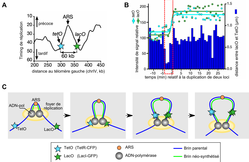
FIGURE 23 – Coordination de deux fourches de réplication au sein du même foyer de réplication. A- Afin de visualiser la progression de deux fourches sœurs, des opérateurs Lac ( LacO ) et Tet ( TetO ) ont été insérés chez la levure de part et d'autre d'une origine de réplication (ARS). Ces deux opérateurs sont visualisés grâce à l'expression des protéines LacI-GFP et TetR-CFP. B- TetO et LacO colocalisent juste avant leur réplication. La fluorescence des spots GFP et CFP est mesurée au cours du temps ; le doublement de la fluorescence correspond au moment où ces loci sont dupliqués par le passage de la fourche de réplication. La distance entre les deux spots est également mesurée : juste avant leur réplication, TetO et LacO colocalisent. C- Modèle explicatif : les deux fourches sœurs émanant de l'origine (ARS) centrale sont fixées dans la même usine de réplication, conduisant à la colocalisation de TetO et LacO lorsqu'ils sont répliqués. Ces figures sont issues et adaptées de Kitamura, E., Blow, J. J., and Tanaka, T. U. (2006). Live-cell imaging reveals replication of individual replicons in eukaryotic replication factories. Cell , 125(7):1297–1308, copyright 2006, avec l'autorisation d'Elsevier.
