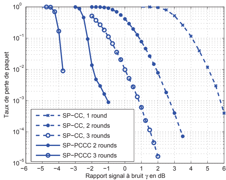
Figure 4.10 — Taux d'erreur paquet pour différents schémas HARQ-SP, dans le cas d'une transmission QPSK sur un canal BABG complexe, avec M_1 = 2 , D = 1024 bits, et H = 40 bits.
