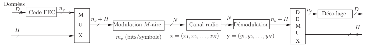
Figure 1.2 — Traitements mis en œuvre par la couche PHY. Noter le codage séparé de l'entête, puis le multiplexage avec les données codées, avant l'opération de modulation proprement dite
