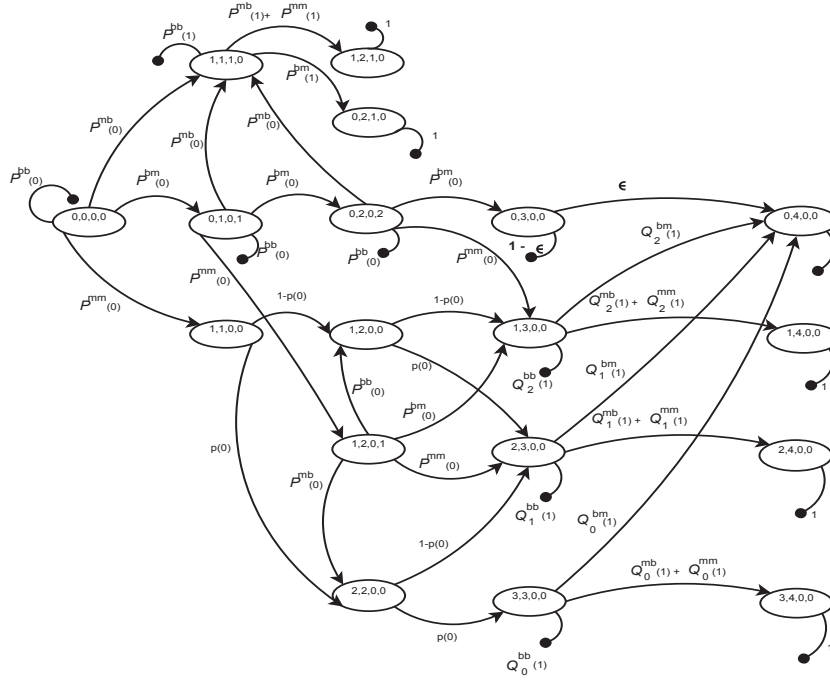
Figure 5.5 — Chaîne de Markov représentant un schéma H-SP-MP pour L = 3 , M_1 = 2 et M_2 = 2 .
