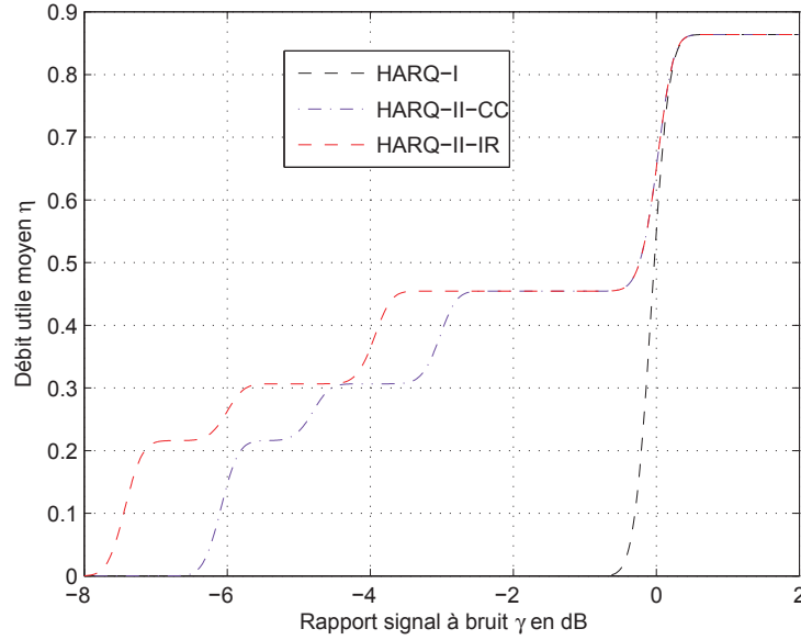
Figure 3.14 — Débit utile en HARQ-I, HARQ-II-CC et HARQ-II-IR pour une transmission sur canal BABG complexe avec des codes optimaux de longueur finie et rendement R_o = 0,96 bits/symbole, M_1 = 3 , D = 512 bits, H = 40 bits et une probabilité de perte \epsilon = 0,1 sur la voie retour
