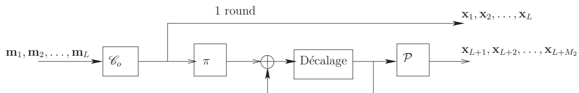
Figure 4.7 — Schéma HARQ-MP basé sur une concaténation série d'un code convolutif et d'un accumulateur (MP-SCCA)
