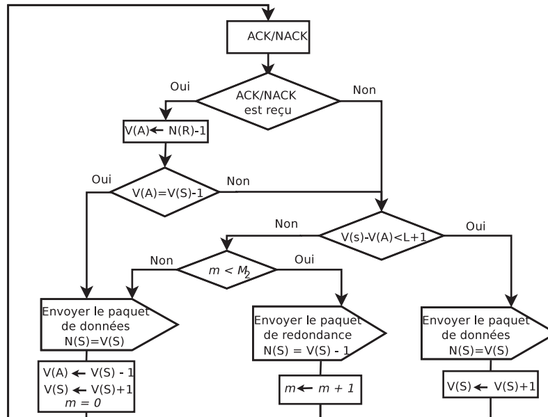
Figure 4.15 — Automate à l'émission de la variante MP-Acq par paquet ( V(A) variable interne contenant le numéro de séquence du dernier paquet positivement acquitté, N(S) numéro de séquence du paquet en cours, V(S) numéro de séquence du prochain paquet à envoyer, N(R) numéro de séquence porté par l'acquittement reçu)
