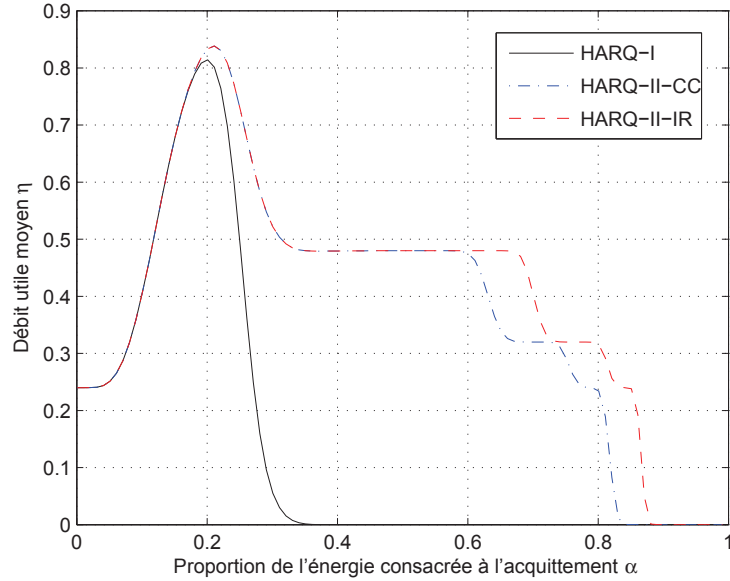
Figure 3.18 — Débit utile pour une transmission HARQ-II-IR avec codes optimaux de longueur finie sur canal BABG réel en fonction de \alpha , pour D = 512 bits, H = 40 bits, R_o = 0,96 bits/symbole, M_1 = 3 , et E_g/N_o = 1 dB
