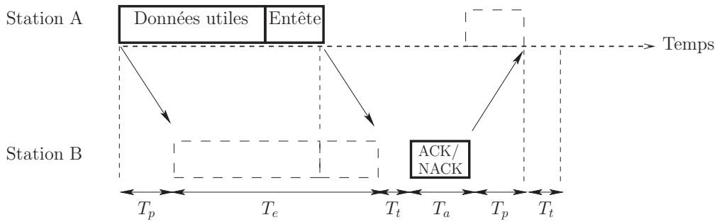
Figure 2.8 — Schéma explicatif montrant les durées d'émission de paquets et d'acquittements, les durées de traitement et le délai de propagation.
