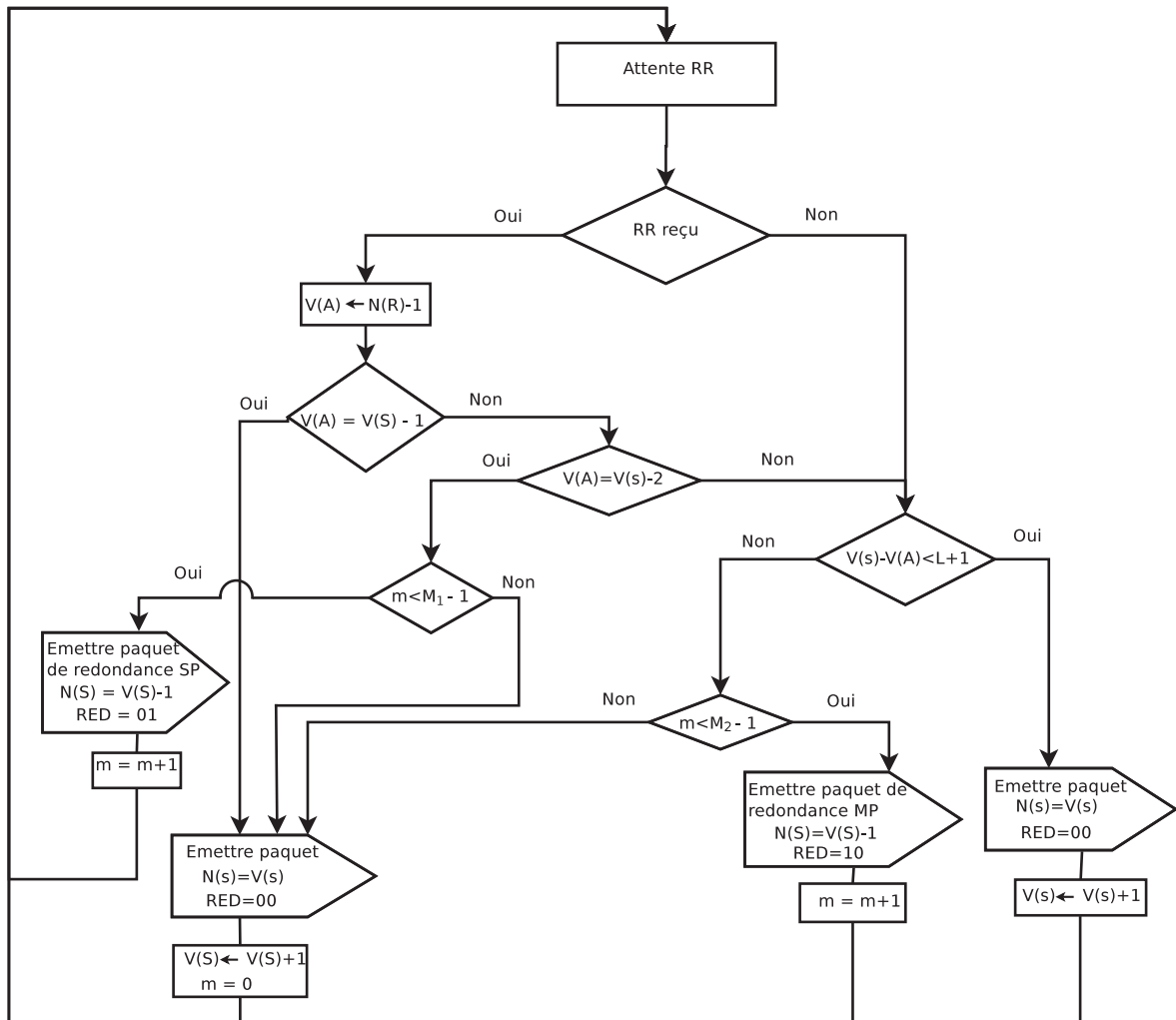
Figure 5.1 — Automate à l'émission du protocole H-SP-MP
