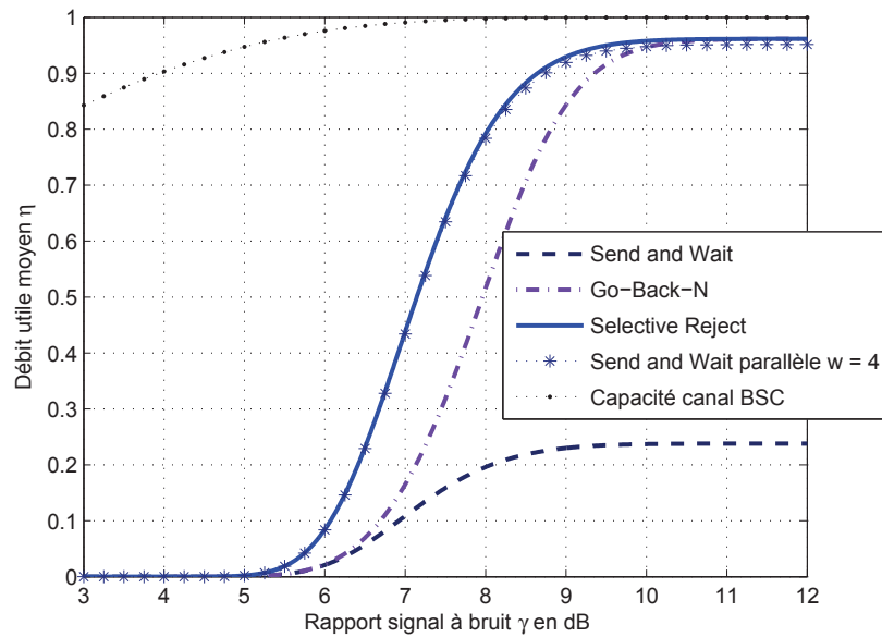
Figure 2.10 — Débit utile normalisé en fonction du RSB en SaW, GBN, SR et PSW pour D = 1000 bits, H = 40 bits et \tau = 3/2 .
