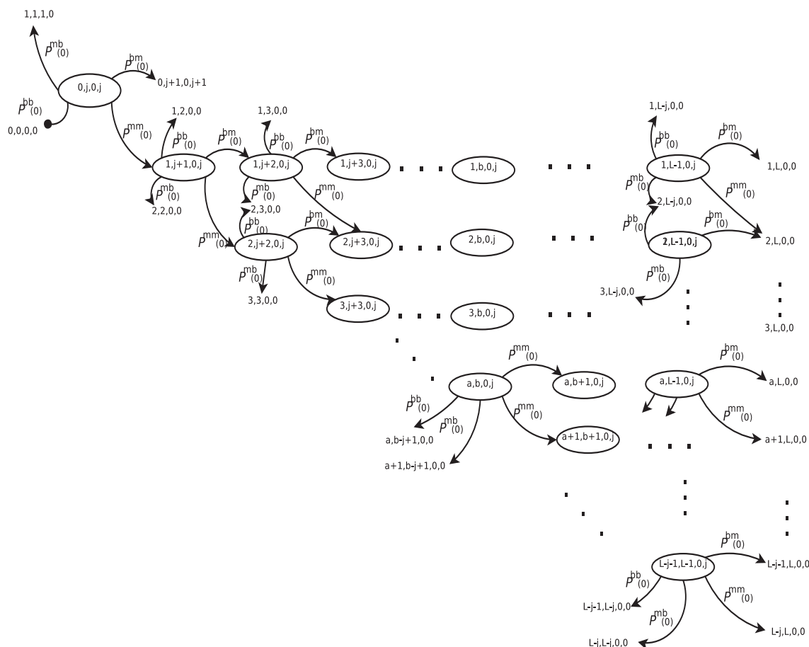
Figure 5.4 — Figure complémentaire de la structure générale de chaîne de Markov de la figure 5.3 représentant les états du mode indéterminé du protocole hybride SP et MP avec paramètres M_1 , M_2 , L . L'état (0, j, 0, j) vérifie 0 < j < L .
