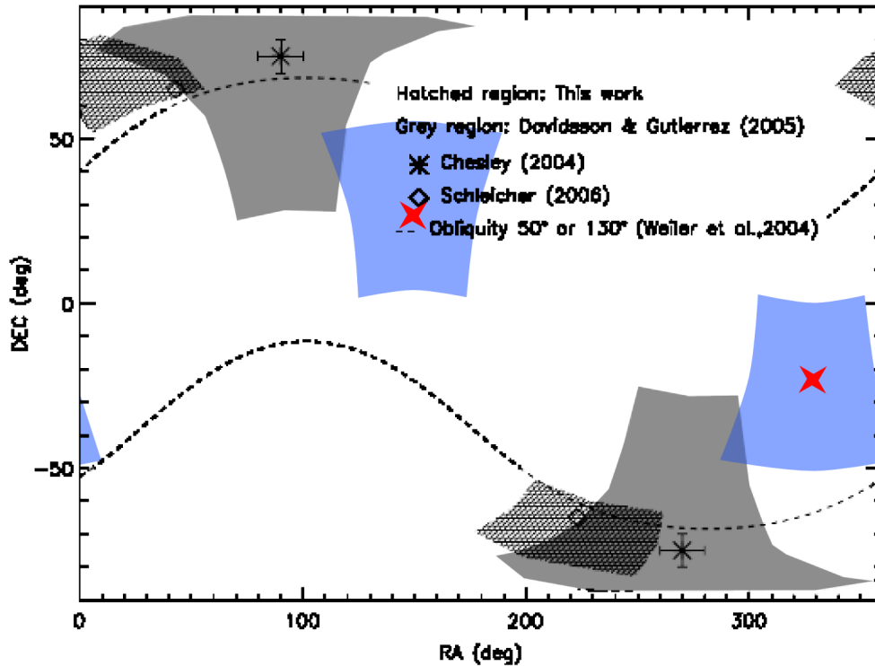
Figure 13.3 – Directions possibles de l’axe de rotation de la comète 67P/Churyumov-Gerasimenko par différents auteurs (Lamy et al., 2007). La croix jaune correspond à notre détermination avec son erreur associée (rectangle bleu).
