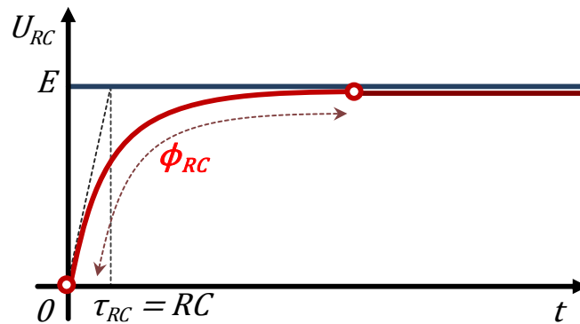
Figure IV-1 : Réponse en tension d'un circuit R//C
