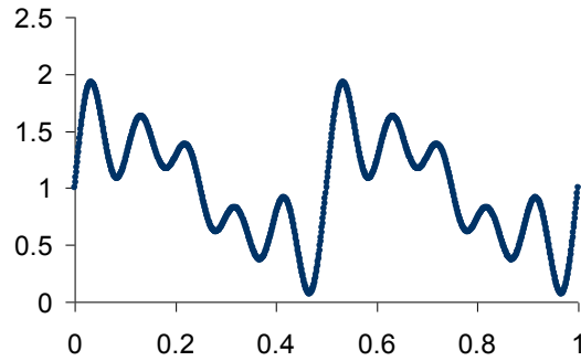
Figure I-44: Exemple de signal "multisine" 5 harmoniques, de fréquence fondamentale 1Hz
