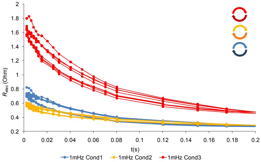
Figure II-52 : Réponse fort signal de R_{elec} à 1mHz, Cond1, Cond2, Cond3
