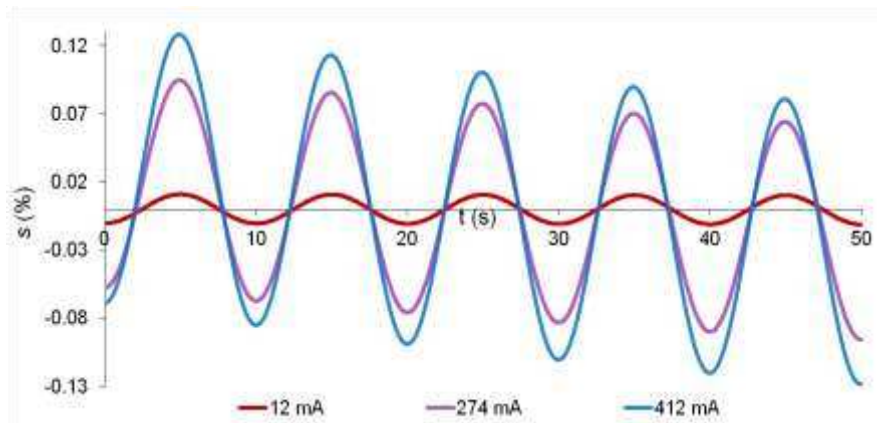
Figure V-11 : Réponse calculée de s à des courant PS à 100mHz ( \langle T_{FC}^{th} \rangle = T_a = 30^\circ C ; HR_a = 70\% )
