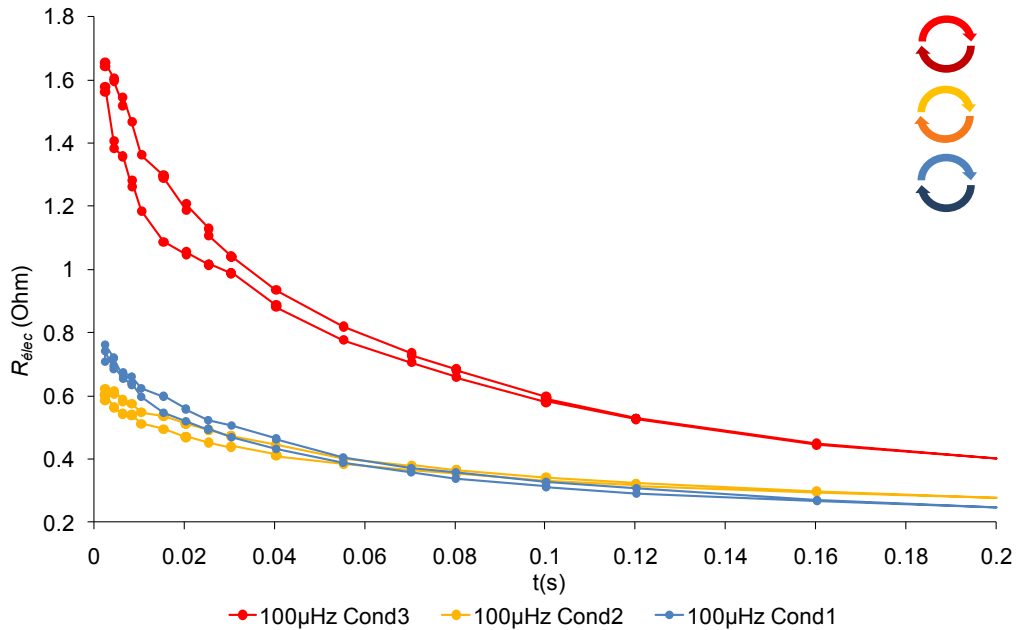
Figure II-54 : Réponse fort signal de R_{élec} à 100μHz, Cond1, Cond2, Cond3
