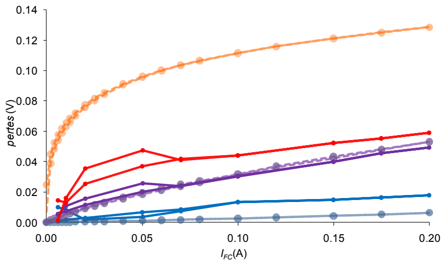
Figure IV-25 : Comparaison des pertes QS extraites via les modèles QS et PS ; Cond1
