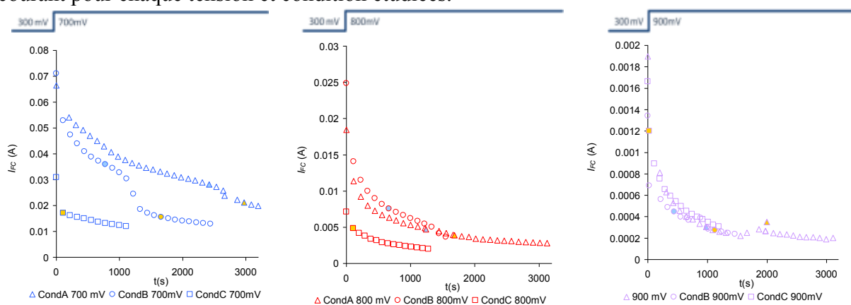
Figure A-9 : Réponses en courant à 700mV, 800mV, 900mV, à CondA, CondB, et CondC
