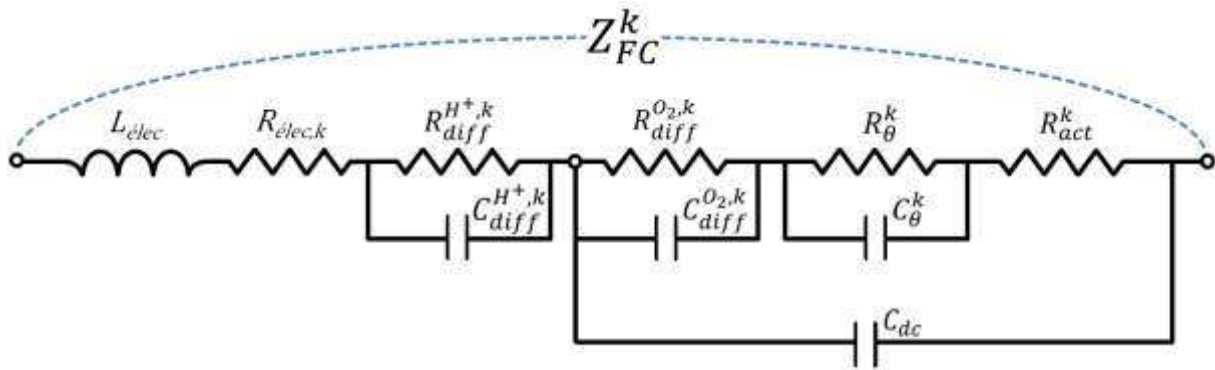
Figure IV-5: Visualisation circuit du modèle d'impédance END de Z^k_{FC} (PNE=1)
