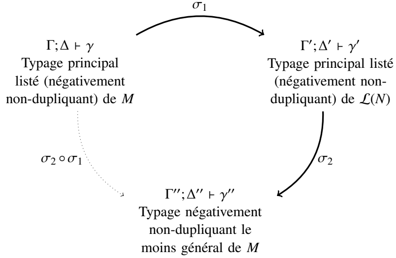
FIG. 5.7 – Relations de typage pour l'analyse dans les ACGs du second ordre
