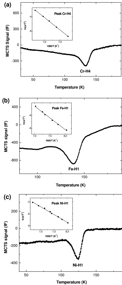
Fig.S.5. Spectres MCTS d'échantillons n -Ge contaminés (a) Cr, (b) Fe, ou (c) Ni. Les mesures ont été effectuées à une polarisation de -5V, durée de pulse optique de 5 ms et une fenêtre de 80 s -1 . L'encart montre la signature du niveau TM-H1.
