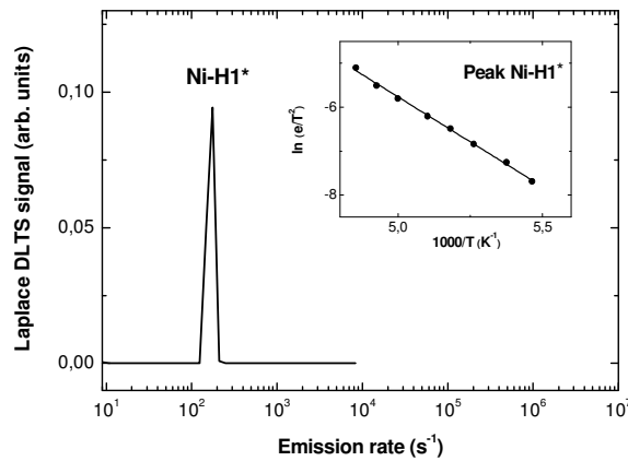
Fig.S.8. Spectre de Laplace DLTS pour un échantillon de p-Ge. Les paramètres d'analyse sont : t_F = 200 \text{ }\mu\text{s} , polarisation (-5V, -2V) et T = 200 \text{ K} . L'encart montre la signature du piège à trou Ni-H1*.
