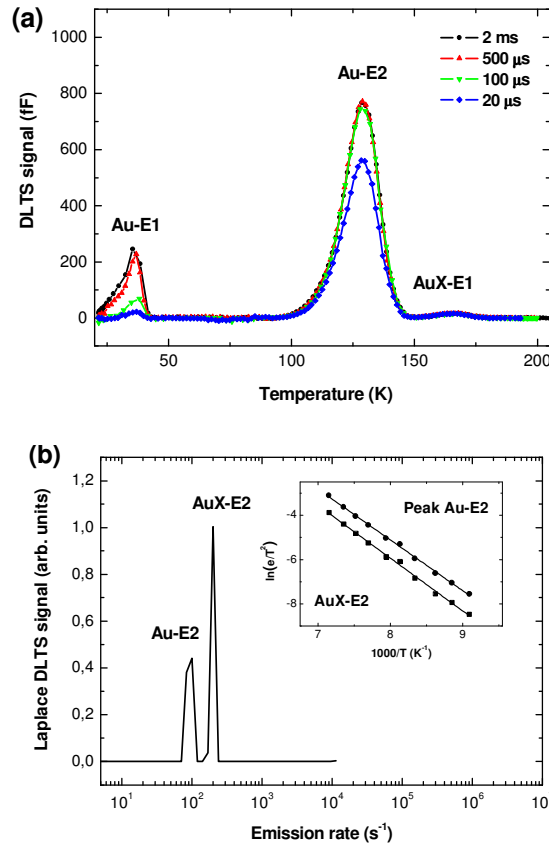
Fig. S.3. Spectre de DLTS (a) et de Laplace DLTS (b) des échantillons n -Ge contaminés avec Au. Les paramètres d'analyse sont les suivant : t_F = 200 \mu s , séquence de pulse (-5V, -2V) , (a) avec une fenêtre de 100 s^{-1} et (b) à T = 130K . L'encart montre la signature des niveaux Au-E2 and AuX-E2.
