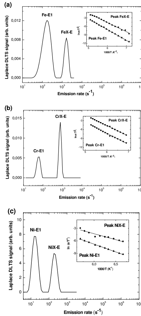
Fig. S.1. Spectres de Laplace DLTS enregistrés dans n -Ge contaminés avec Fe (a), Cr (b) ou Ni (c). Les paramètres d'analyse sont les suivant : t_F = 200 \mu s pour tous les, (a) séquence de pulse (-4V, -2V) et T = 180K ; (b) séquence de pulse (-4V, -1.5V) et T = 175K ; (c) séquence de pulse (-5V, -2V) et T = 180K . L'encart montre les signatures des niveaux TM-E1 and TMX-E.
