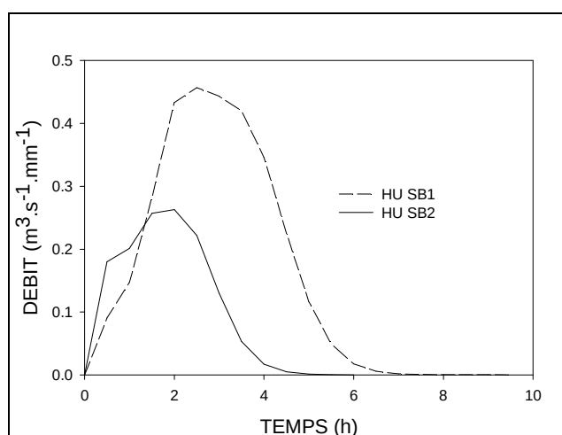
Figure II. 12 – Hydrogrammes unitaires à ½ heure pour les sous-bassins SB1 et SB2 obtenu avec RuiCell.
