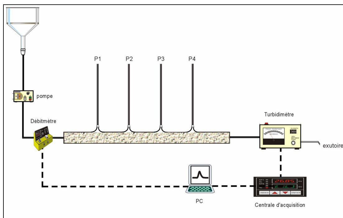
Figure IV. 2 – Dispositif expérimental.
