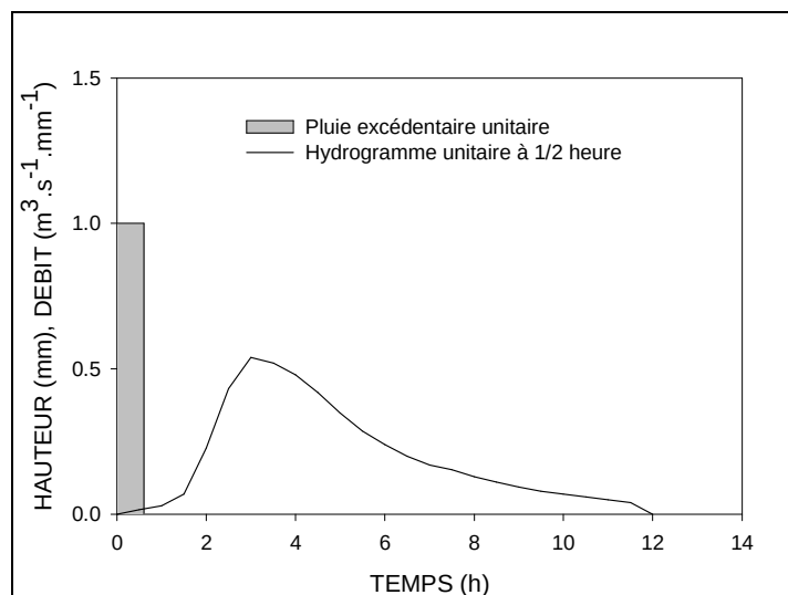
Figure II. 7 – Hydrogramme unitaire à ½ heure HU_{0,5} calculé par déconvolution (modèle global).
