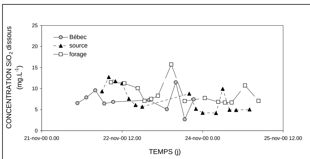
Figure III. 63 – Evolution de SiO₂ en solution à la perte, à la source et au forage (novembre 2000).
