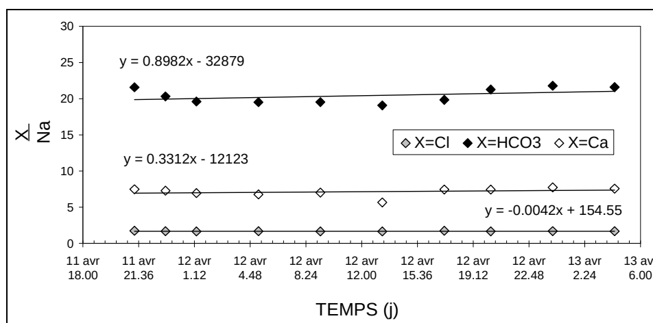
Figure III. 69 – Evolution des concentrations en \text{HCO}_3 et Ca comparée à celle d'une espèce conservative (Cl) au cours de la crue d'avril 2000.
