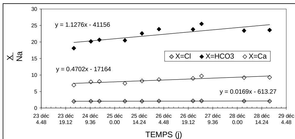
Figure III. 68 – Evolution des concentrations en \text{HCO}_3 et Ca comparée à celle d'une espèce conservative (Cl) au cours de la crue de décembre 1999.
