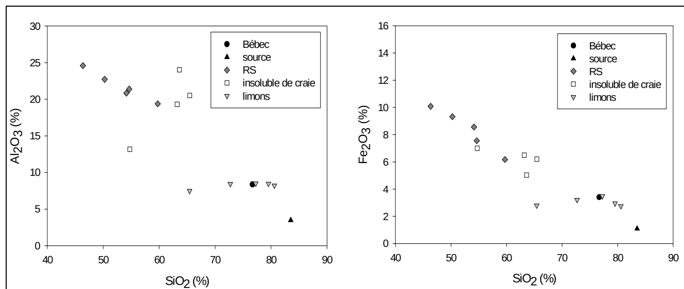
Figure III. 50 – Teneurs en silice par rapport à l'alumine.
