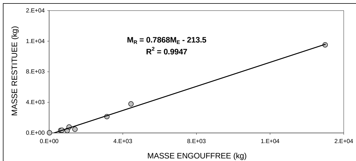
Figure III. 66 – Relation linéaire entre la masse engouffrée et la masse restituée à la source.
