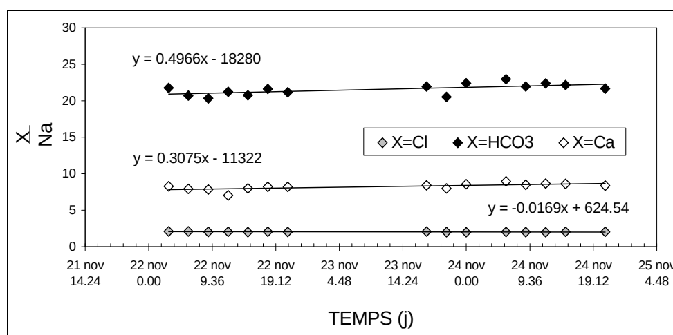
Figure III. 70 – Evolution des concentrations en \text{HCO}_3 et Ca comparée à celle d'une espèce conservative (Cl) au cours des crues de novembre 2000.
