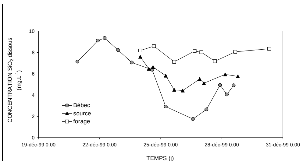
Figure III. 57 – Evolution de \text{SiO}_2 en solution à la perte, à la source et au forage (décembre 1999).
