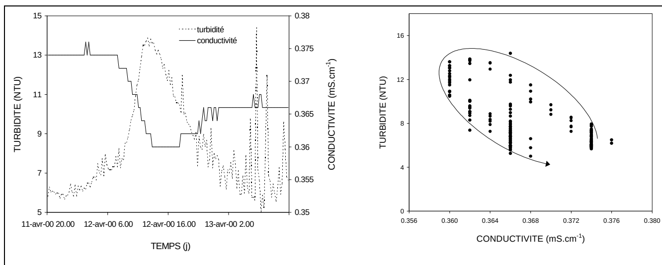
Figure III. 20 – Evolution de la turbidité et de la conductivité électrique à la source au cours de la crue du 12 avril 2000.
