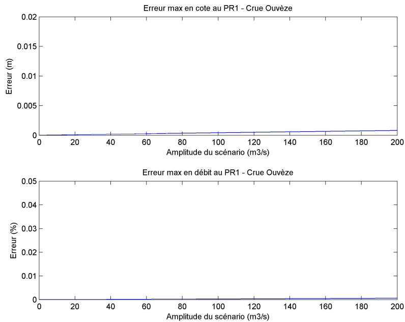
FIGURE B.12 – Évolution de la différence en débit et en cote entre le modèle linéaire et le modèle non-linéaire au PR1 pour différents échelons de débit à l'Ouvèze
