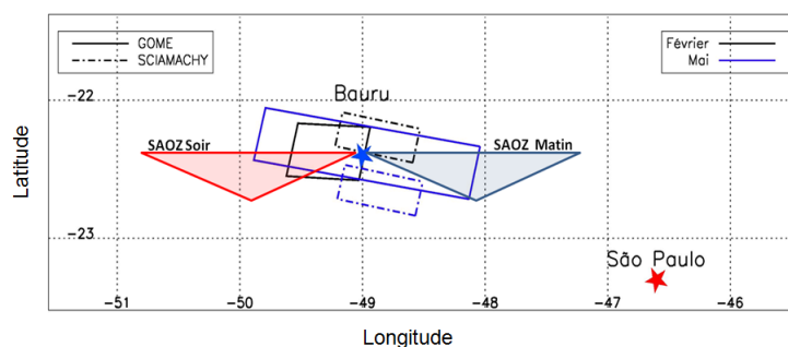
FIGURE 2.4 – Comparaison des mailles d'observation des instruments : GOME, SCIAMACHY et SAOZ à Bauru
