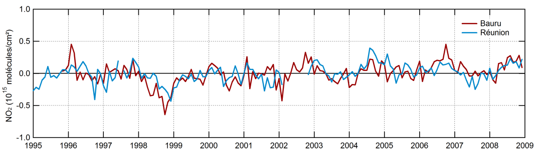
FIGURE 1.3 – Anomalies de NO 2 à Bauru (courbe rouge) et à La Réunion (courbe bleue), observées par les SAOZ.
