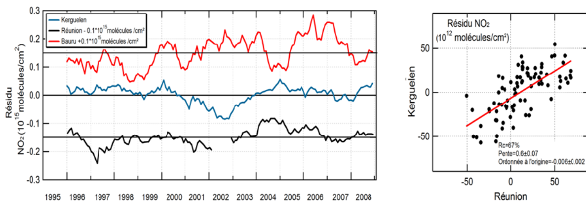
FIGURE 3.9 – Gauche : Variations résiduelles de NO 2 à Bauru (rouge), à La Réunion (noir) et Kerguelen (bleu). Pour plus de visibilité, les courbes ont été décalées de 0.1 \cdot 10^{15} molécules/cm 2 . Droite : corrélation entre les résidus de NO 2 à Kerguelen et La Réunion entre 2001 et 2008.
