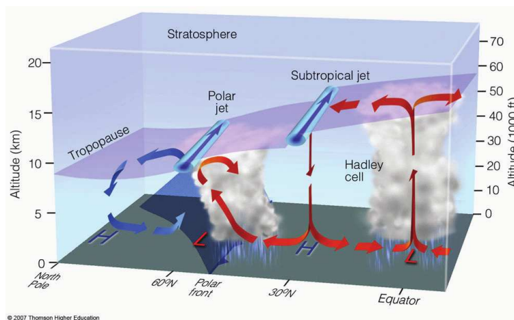
FIGURE 2.5 – Coupe méridienne des grandes cellules de circulation dans l’Hémisphère Nord. (NRC, 2010)
