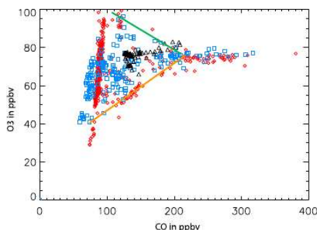
FIGURE 3.7 – Correlations entre rapports de mélange de CO et d’ozone le long du vol du DLR Falcon le 22 juillet 2004, dans les observations in-situ (rouge), simulées par MOCAGE (noir) et reconstruites par ZooM-CiTTY (bleu). Les lignes orange et verte indiquent les lignes de mélange. Source : Real et al. (2010).
