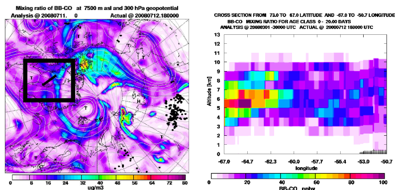
FIGURE 5.1 – Prédiction par le modèle FLEXPART de la distribution du CO issu de feux de biomasse en Arctique le 12 juillet 2008 à 18h UTC. La carte de gauche indique le rapport de mélange à 7.5 km d'altitude et la figure de droite est une coupe verticale du champ de CO à l'Ouest du Groenland. Le rectangle noir indique la zone où a eu lieu l'expérience PERTRAS, et les points noirs indiquent la localisation des feux boréaux. (Source : A. Stohl, NILU)
