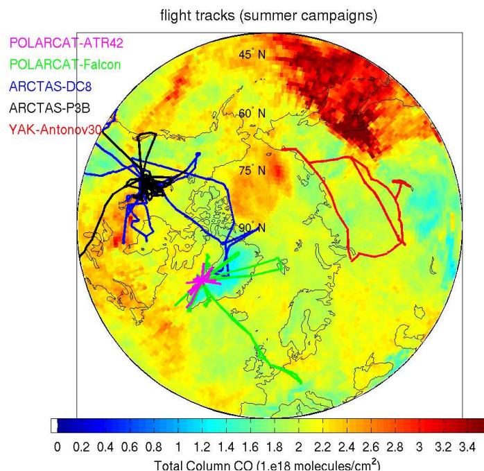
FIGURE 2.11 – Carte des colonnes de CO moyennes durant la campagne d’été au-dessus de l’Arctique mesurées par l’instrument IASI. Les plans de vol de différents avions de recherche pendant la campagne d’été y sont indiqués par les lignes de couleur. Source : Pommier et al. (2010)
