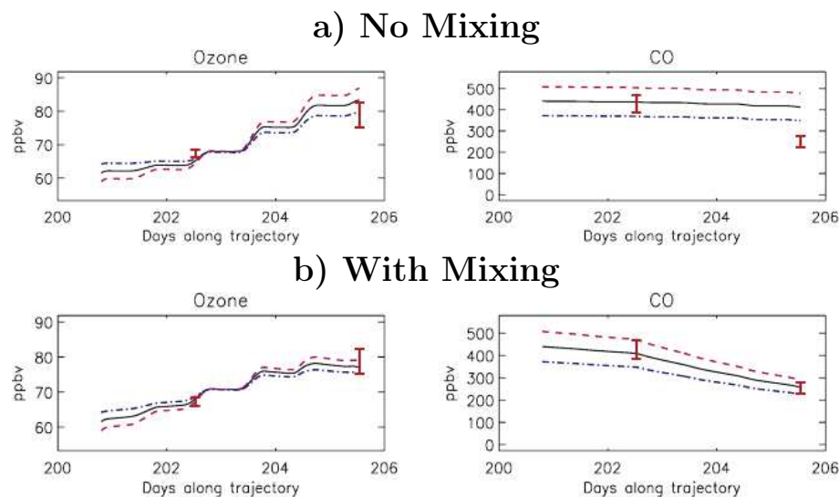
FIGURE 3.2 – Rapports de mélange en ozone et CO simulés dans un panache issu de feux de forêt en Alaska lors de son transport dans la troposphère libre au-dessus de l’Atlantique Nord. Les simulations ont été effectuées avec le modèle CiTTyCAT sans (a) et avec (b) mélange. Source : Real et al. (2007).
