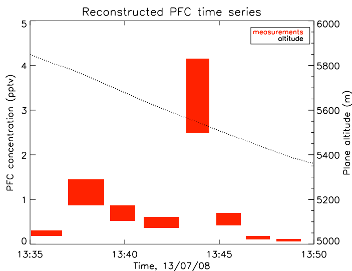
FIGURE 5.5 – Série temporelle des mesures de traceur PFC effectuées le 13 juillet par le DLR Falcon dans le cadre de l’expérience PERTRAS. Les mesures sont présentées sous forme de rectangles dont la largeur correspond à la durée de prélèvement de l’échantillon, et la hauteur aux incertitudes de mesure. L’altitude de l’avion est indiquée par les pointillés noirs.
