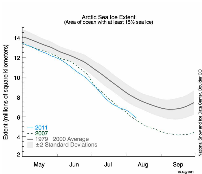
FIGURE 2.9 – Evolution saisonnière de la superficie de la glace de mer en Arctique pour les années 1979-2000 (gris, avec enveloppe correspondant au double écart-type), 2007 (vert) et 2011 (bleu). Source : site web du NSIDC, http://nsidc.org/arctocsseaicnews
