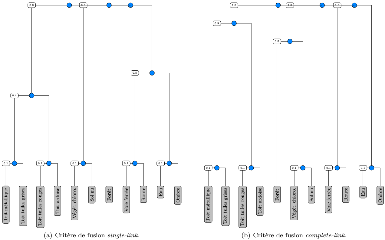
FIGURE 12.2 – Dendrogrammes associés à la matrice de dissimilarité présentée dans la table 12.2. Les instances initiales sont représentées par des rectangles gris tandis que les instances de plus hauts niveaux sémantiques sont représentées par des disques bleus.
