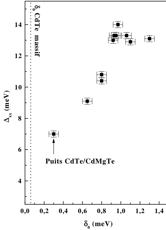
Figure 5.8 – Energie de liaison du biexciton pour différentes boîtes quantiques, en fonction du dédoublement d'échange \delta_0 .
