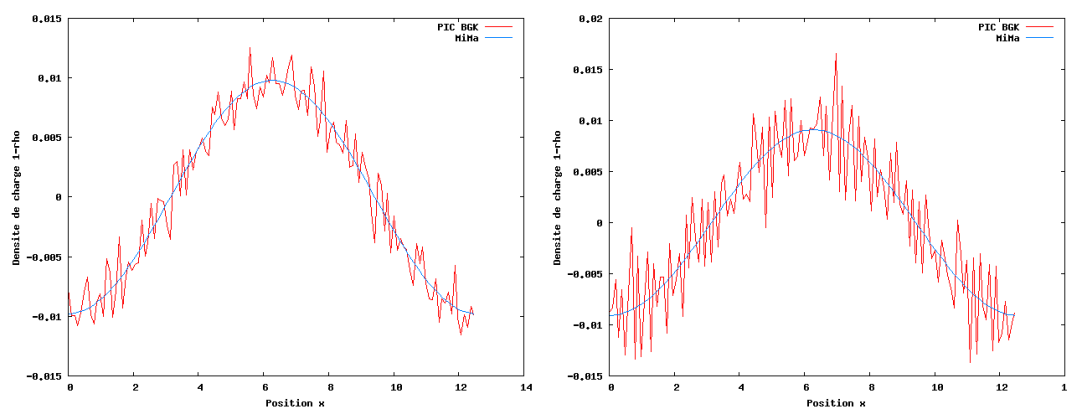
FIGURE 5.6 – Test 1, \varepsilon = 1 - Densité de charge ( 1 - \rho ) aux temps t = 0.2 (à gauche) et t = 0.4 (à droite), pour PIC-BGK (en rouge) et MiMa (en bleu) avec N_p = 5 \times 10^5 .
