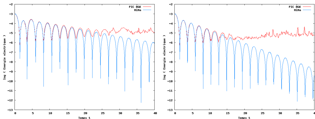
FIGURE 5.4 – Test 1 - Énergie électrique au cours du temps : MiMa (en bleu) et PIC-BGK (en rouge) avec N_p = 5 \times 10^5 , pour \varepsilon = 1 (à gauche) et \varepsilon = 10 (à droite).
