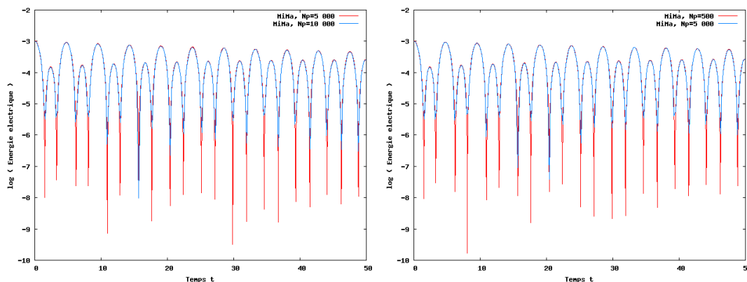
FIGURE 5.18 – Test 1 - Nombre de particules nécessaires pour \varepsilon = 10^{-2} (à gauche) et \varepsilon = 10^{-5} (à droite).
