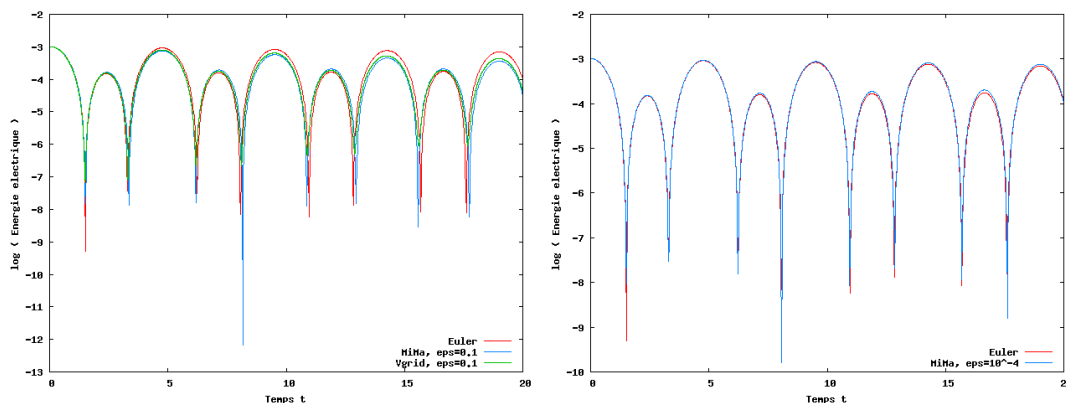
FIGURE 5.2 – Test 1 - Énergie électrique au cours du temps : MiMa avec N_p = 5 \times 10^3 (en bleu) comparé à Euler (en rouge) et Vlasov-Poisson sur grille (en vert) pour \epsilon = 0.1 (à gauche) et \epsilon = 10^{-4} (à droite).
