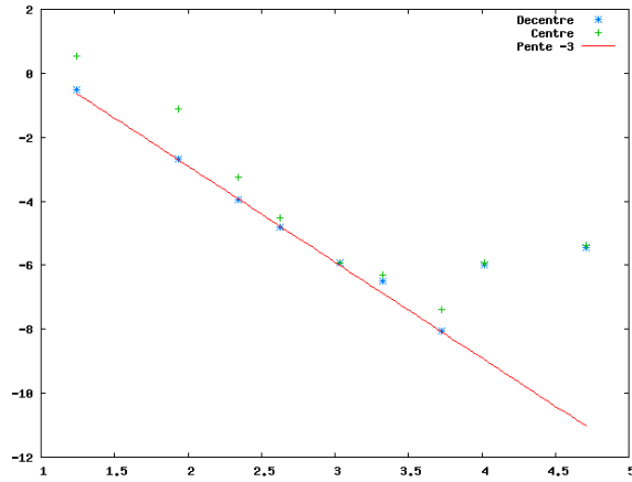
FIGURE 7.8 – Onde plane (7.133) dans un disque - Erreur sur \phi en norme L2 au temps t = 1 pour un flux décentré (en bleu) et centré (en vert), échelle logarithmique dans les deux directions, pente -3 en rouge.
