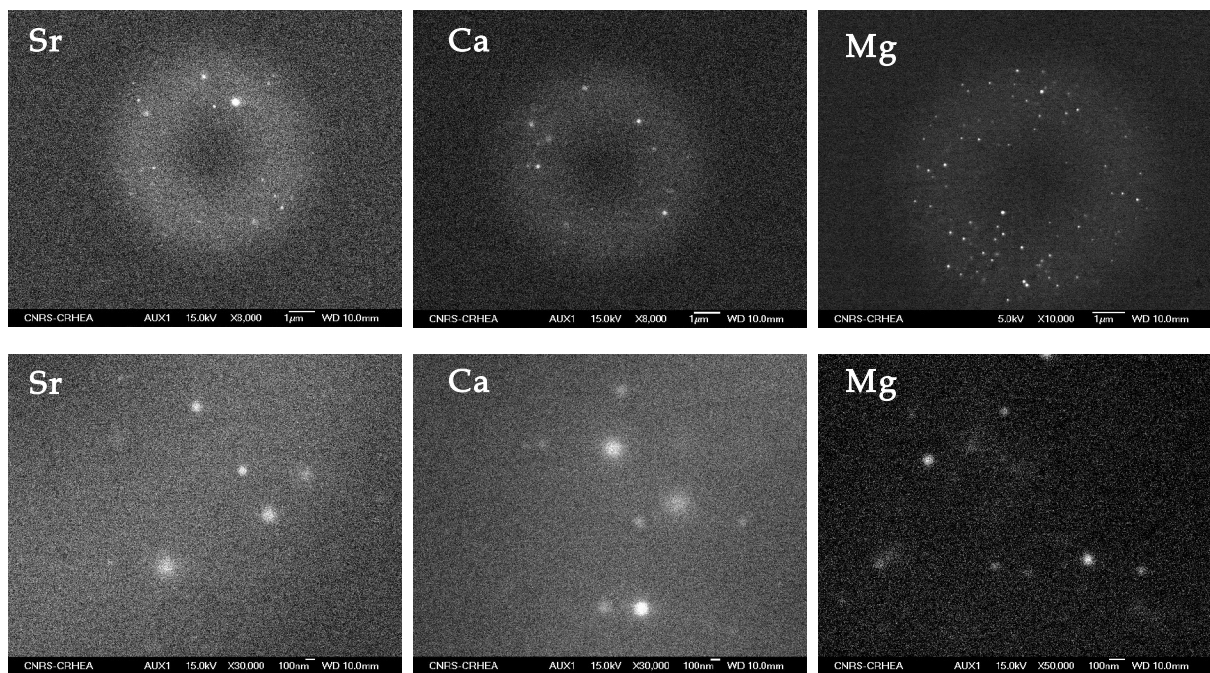
Figure IV.3: Images par Microscopie Électronique à Balayage de fibres clivées transversalement. La concentration en ions de terre alcaline dans la solution est 0,1 \text{ mol/l} .
