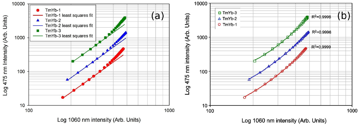
Figure III.8: Représentation log/log de la fluorescence à 475 nm de Tm^{3+} en fonction de la luminescence à 1060 nm de Yb^{3+} , pour une puissance de pompe incidente comprise entre 3 et 108 mW. Les mesures sont décalées en ordonnée pour aider à la comparaison. L'ajustement a été réalisé sans ESA (a) et avec ESA (b).
