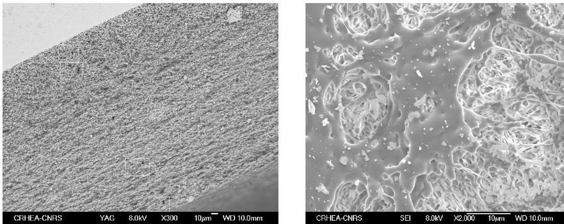
Figure II.11 : gauche : Image par Microscopie Électronique à Balayage d'une coupe transversale d'une couche poreuse déposée par MCVD sur un tube substrat de silice. L'échantillon est « clivé » transversalement. Droite : Image par Microscopie Électronique à Balayage d'une couche poreuse vue du dessus.
