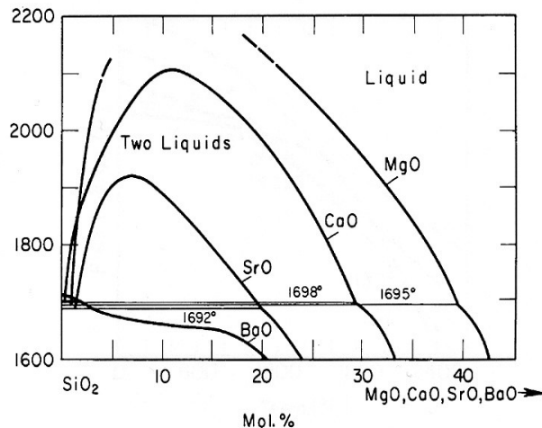
Figure IV.2: Diagrammes de phase des binaires \text{SiO}_2\text{-MO} ( M=\text{Sr}, \text{Ca}, \text{Mg} ).
