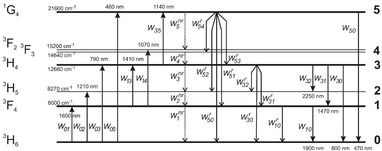
Figure III.1 : Diagramme énergétique de \text{Tm}^{3+} . Les paramètres sont présentés dans le texte.
