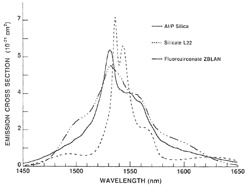
Figure II.5 : Spectres de sections efficaces d'émission de Er^{3+} dans différents verres. (figure extraite de 4)
