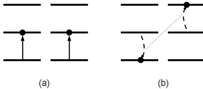
Figure II.7 : Représentation du mécanisme de transfert d'énergie par up-conversion .
