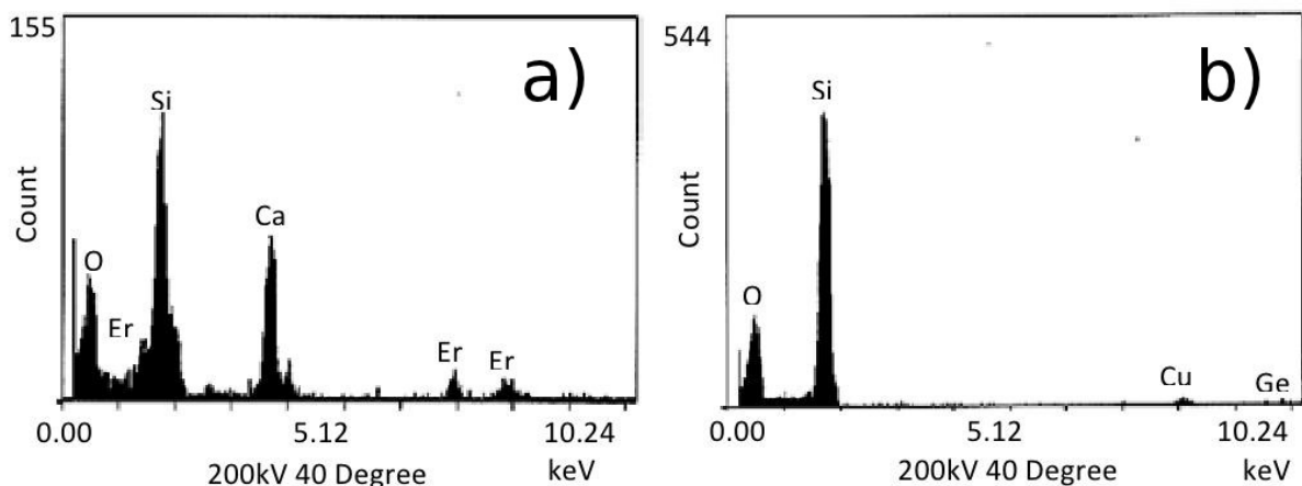
Figure IV.5 : Mesures de la composition par EDX dans un cœur de préforme. Le faisceau est pointé (a) sur ou (b) en dehors d'une particule.
