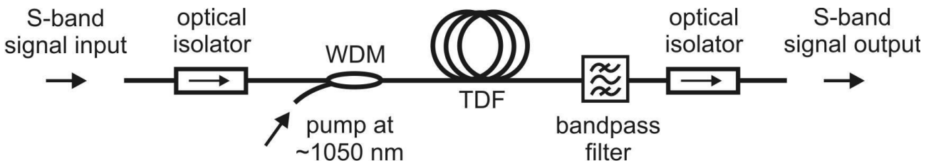
Figure III.9: Exemple de montage pour un dispositif à base de fibre amplificatrice à 1,47 µm.
