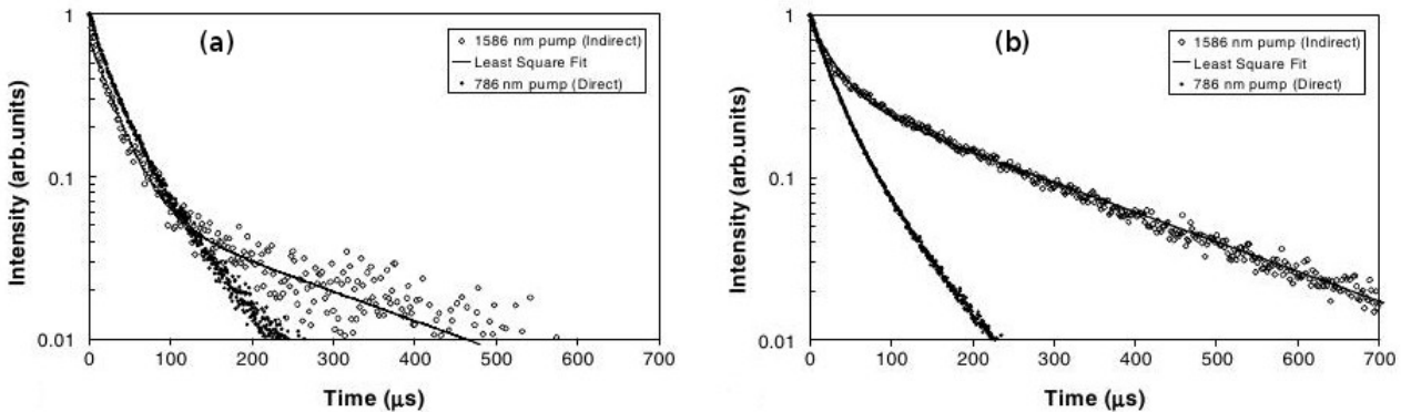
Figure III.6: Déclinés de fluorescence à 800 nm pour une excitation à 786 et 1586 nm dans une fibre dopée Tm^{3+} . La concentration en Tm_2O_3 est de 200 (a) et 2900 (b) ppm mol.
