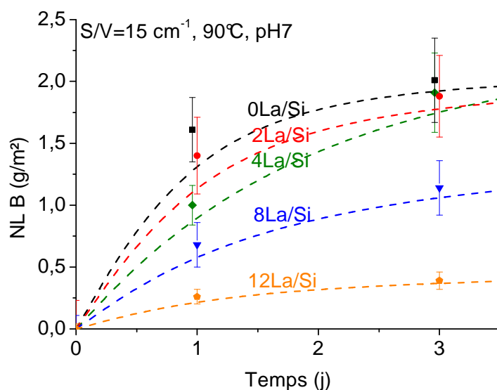
Figure 97. Pertes de masses normalisées en bore aux premières échéances à pH7 pour les verres à teneurs variables en oxyde de lanthane (série x\text{La/Si} , 90^\circ\text{C} , S/V=15\text{ cm}^{-1} ) - Les pointillés servent de guide visuel
