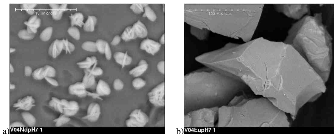
Figure 95. Clichés MEB des verres altérés en mode dynamique à pH7 et 90°C a) avec 4%mol Nd_2O_3 (zoom sur les précipités), b) avec 4%mol Eu_2O_3
