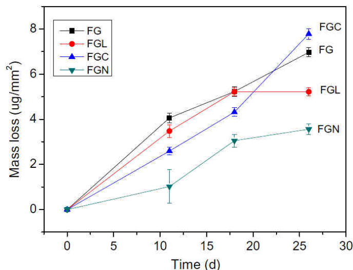
Figure 26. Pertes de masse au cours du temps pour différents verres (FG: sans oxyde de terre rare; FGC: avec 1%mol CeO_2 ; FGL: avec 1%mol La_2O_3 et FGN: avec 1%mol Nd_2O_3 ) dans une solution alcaline et à température ambiante, d'après [Wang et al., 2010]
