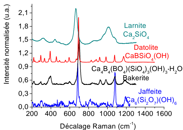
Figure 125. Spectres Raman de silicates de calcium, d'après [Rruff]
