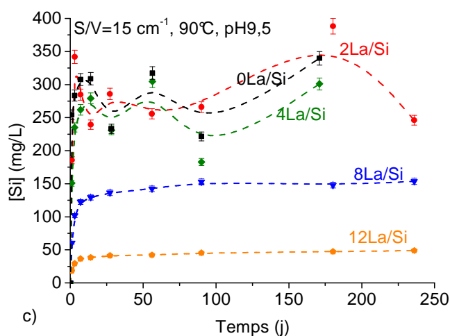
Figure 105. Pertes de masses normalisées en bore (a) et en sodium (b), concentration en silicium (c) au cours du temps pour une altération à pH9,5, à 90°C avec un S/V=15 \text{ cm}^{-1} pour la série de verres riches en oxyde de lanthane ( x\text{La/Si} ) - Les pointillés servent de guide visuel
