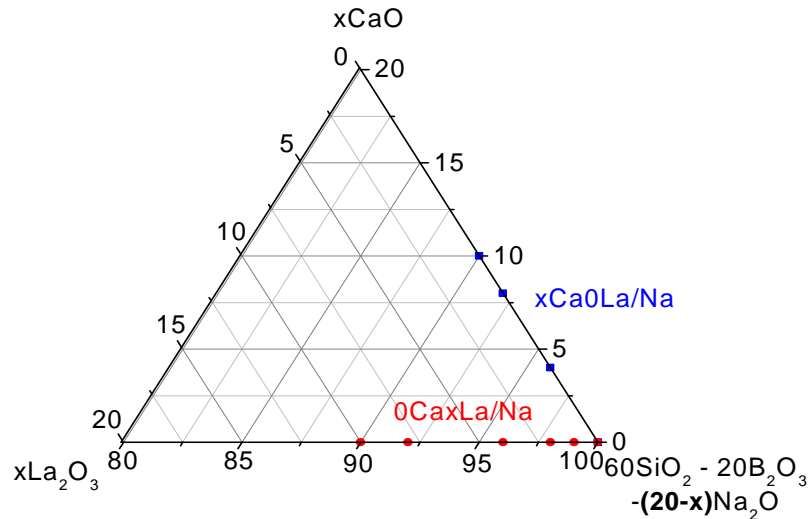
Figure 37. Zoom sur le diagramme ternaire (%mol) représentant les compositions des deux séries de verres 0\text{CaxLa}/\text{Na} et x\text{Ca}0\text{La}/\text{Na}
