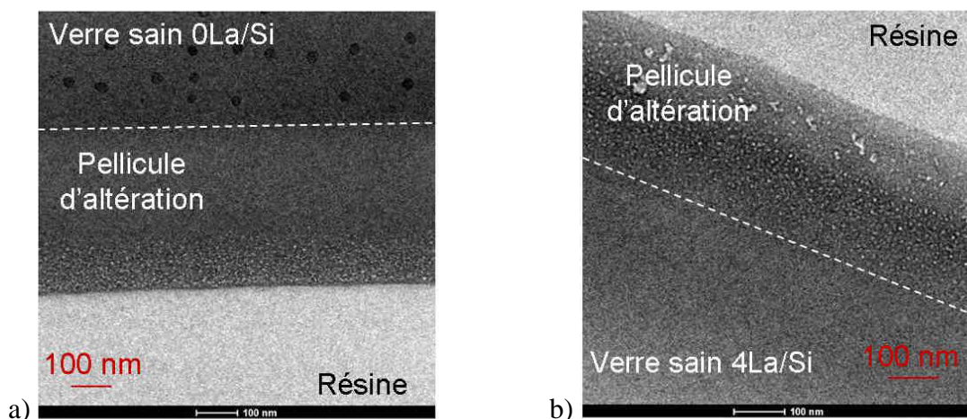
Figure 133. Clichés MET de coupes FIB de verres altérés à pH7 et à 90°C pendant 90 jours (a) verre sans terre rare et b) verre avec 4%mol La_2O_3 (4La/Si)
