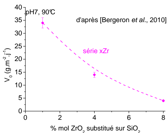
Figure 92. Vitesses initiales de dissolution à \text{pH} 7 et à 90^\circ\text{C} pour des teneurs variables en \text{ZrO}_2 (substitué sur \text{SiO}_2 ), d'après [Bergeron et al. , 2010] - Les pointillés servent de guide visuel
