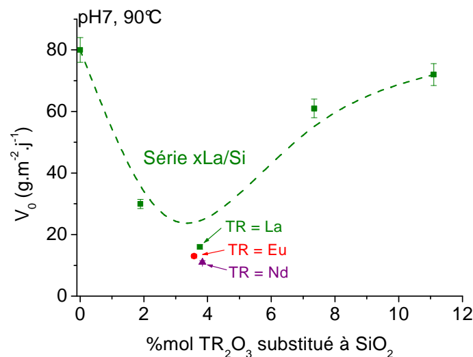
Figure 84. Vitesses initiales de dissolution à pH7 et à 90°C en fonction de la teneur en \text{La}_2\text{O}_3 et pour différentes natures de terres rares (La, Nd et Eu - 4%mol \text{TR}_2\text{O}_3 ) où 1 \text{TR}_2\text{O}_3 substituée à la place de 1 \text{SiO}_2 - Les pointillés servent de guide visuel
