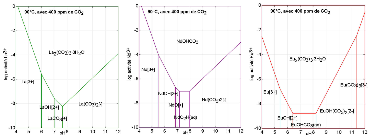
Figure 103. Activité des ions terres rares \text{La}^{3+} , \text{Nd}^{3+} et \text{Eu}^{3+} en fonction du pH et à 90°C pour une teneur en \text{CO}_2 dissous fixée à 400 ppm, d'après [CHESS]
