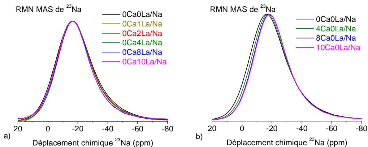
Figure 69. Spectres de RMN MAS de ^{23}\text{Na} pour les séries de verres riches en a) lanthane ( 0\text{Ca}_x\text{La}/\text{Na} ) et b) calcium ( x\text{Ca}0\text{La}/\text{Na} ) – ( x\text{La}_2\text{O}_3 et x\text{CaO} ajoutés à la place de x\text{Na}_2\text{O} )
