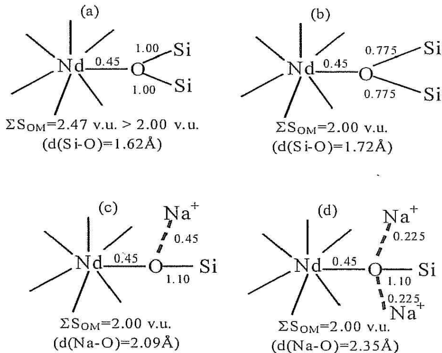
Figure 13. Représentation schématique de la connectivité entre un polyèdre de \text{NdO}_7 et : a) deux atomes de silicium appartenant au réseau silicaté, à travers un atome d'oxygène pontant (BO), (b) deux atomes de silicium appartenant au réseau silicaté, à travers un BO et avec une distance Si-O satisfaisant les règles de stabilité de Pauling, (c) un ion sodium et un atome de silicium appartenant au réseau silicaté, à travers un NBO, (d) deux ions sodium et un atome de silicium appartenant au réseau silicaté, à travers un NBO. Les valeurs indiquées à côté des liaisons correspondent aux valences de liaison, d'après [Caurant et al. , 2009].
