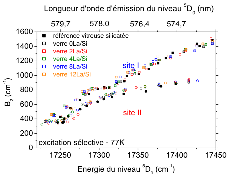
Figure 155. Evolution du paramètre B_2 en fonction de l'énergie d'émission {}^5D_0-{}^7F_0 pour la référence silicatée (■,●) et tous les verres sains de la série en pourcentage croissant en lanthane à 77 K (ronds et carrés vides)
