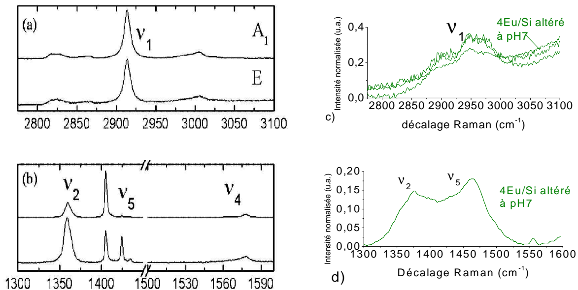
Figure 107. Spectres Raman a-b) des formiates de La (La(HCOO) 3 ) d'après [Silva et al., 2009] et c-d) du verre altéré 4Eu/Si à pH7
