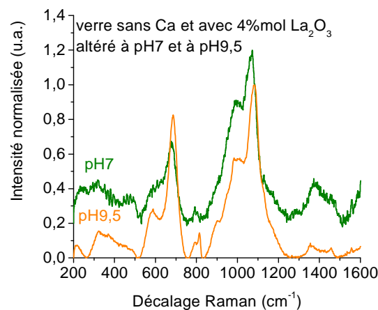
Figure 126. Spectres Raman d'un verre sans oxyde de calcium mais avec 4%mol La_2O_3 altéré à pH7 et à pH9,5
