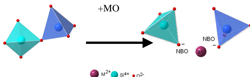
Figure 3. Rupture d'une liaison Si-O-Si et création des atomes d'oxygène non-pontants par ajout d'ions alcalino-terreux ( M^{2+} )
