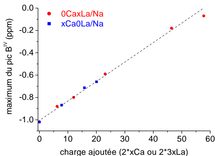
Figure 64. Corrélations entre la position du maximum du pic des atomes de bore tétracoordinnés et la charge ajoutée ( x2 pour 1\text{CaO} et x6 pour 1\text{La}_2\text{O}_3 ) - Les pointillés servent de guide visuel
