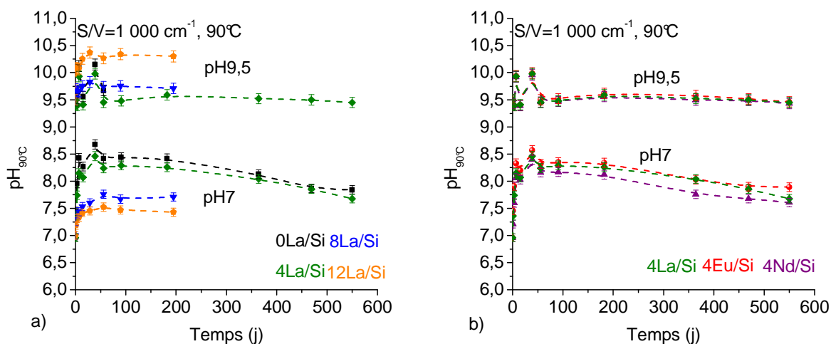
Figure 175. Evolution du pH, mesuré à 90^\circ\text{C} , au cours du temps lors des altérations ( S/V=1000 \text{ cm}^{-1} ) des séries de verre a) à teneur variable en lanthane et b) avec différentes nature de terre rares – Les pointillés servent de guide visuel
