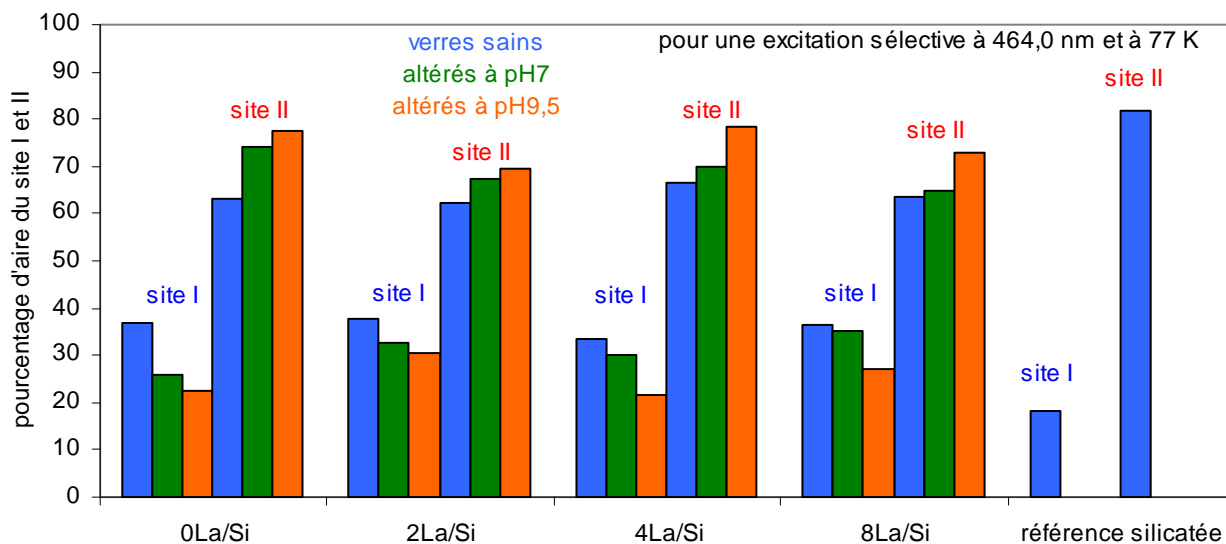
Figure 164. Evolutions des pourcentages des sites I et II déduits à partir de la transition {}^5D_0-{}^7F_0 pour une excitation sélective à 464,0 nm et à 77 K et pour les verres (sains et altérés à pH7 et 9,5) et la référence silicatée
