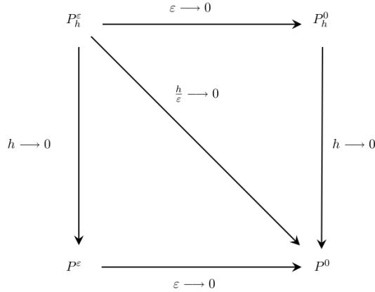
FIGURE 1.1 – Définition des schémas « asymptotic preserving ».
