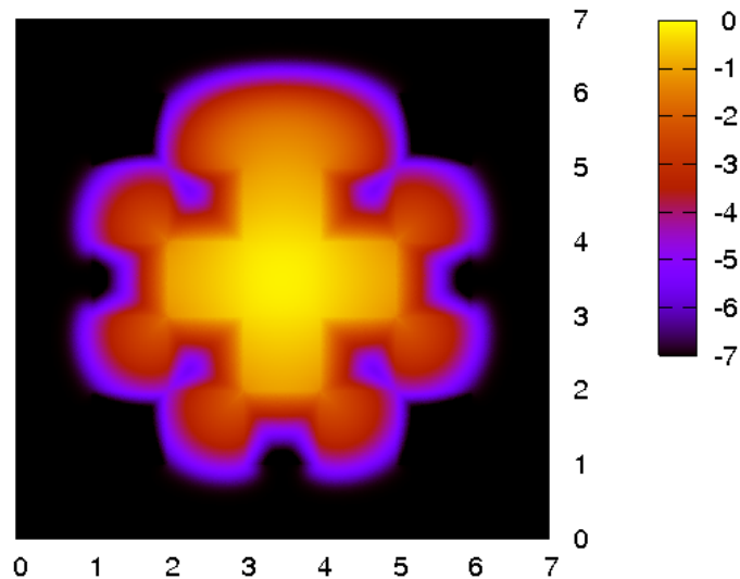
FIGURE 2.17 – Résultat du test sur un maillage 280*280 aléatoire sauf les frontières entre les domaines.
