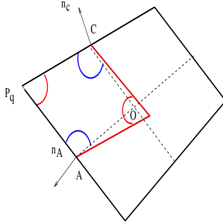
FIGURE 3.4 – Hypothèse du schéma de Breil-Maire
