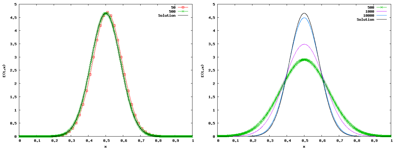
FIGURE 1.4 – À gauche : solutions numériques du schéma de Gosse Toscani avec 50 et 500 mailles, à droite : solutions numériques du schéma upwind avec 500, 1000 et 10000 mailles
