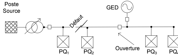
Figure I.7. L'îlotage intentionnel d'une artère du réseau de distribution avec une GED.
