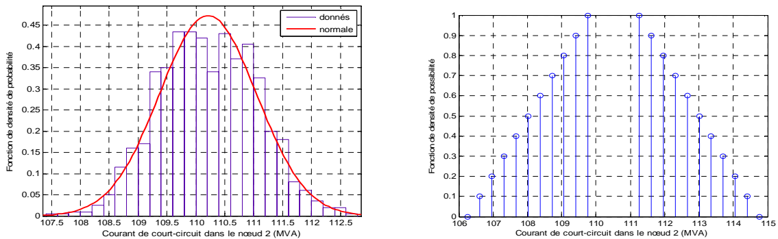
Figure III.28. Puissance de court-circuit biphasé à terre dans le nœud 2 obtenu par (a) la méthode de Monte-Carlo (b) la méthode de l'arithmétique de nombres flous.
