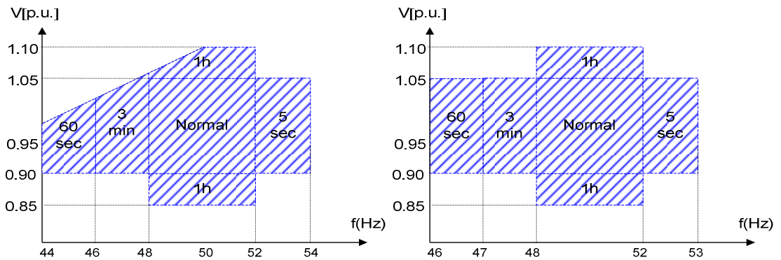
Figure IV.15. Tensions et fréquences des éoliennes du réseau filien française (a) HTB (b) HTA.
