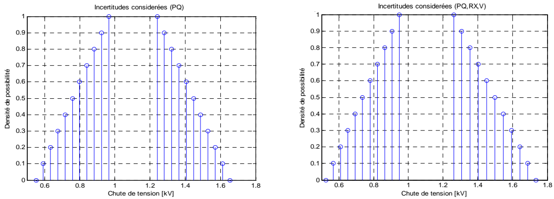
Figure II.6. Chute de tension possibiliste par la méthode de l'arithmétique floue en considérant l'incertitude : (a) de la charge (b) de la charge, ligne et tension du poste source.
