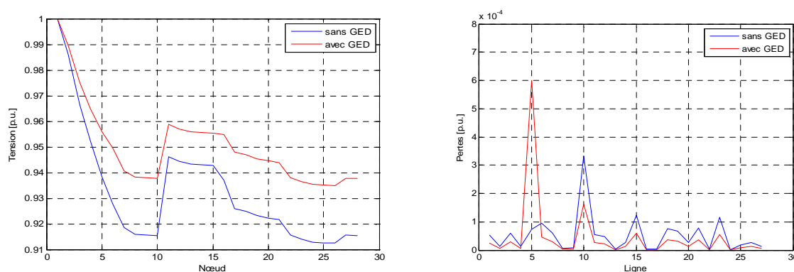
Figure III.13. Profil de tension et de pertes de ligne du réseau 28 bus test.
