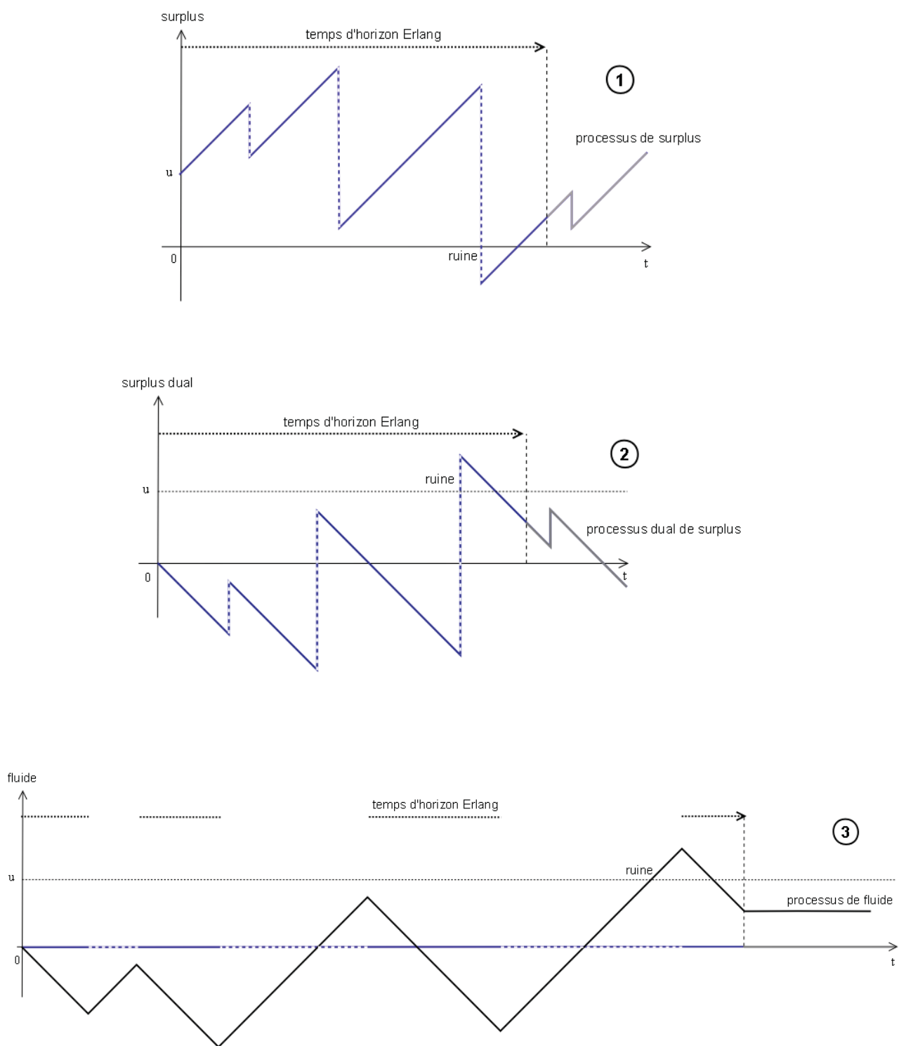
FIGURE 3.1 – Du processus de surplus au processus de fluide
