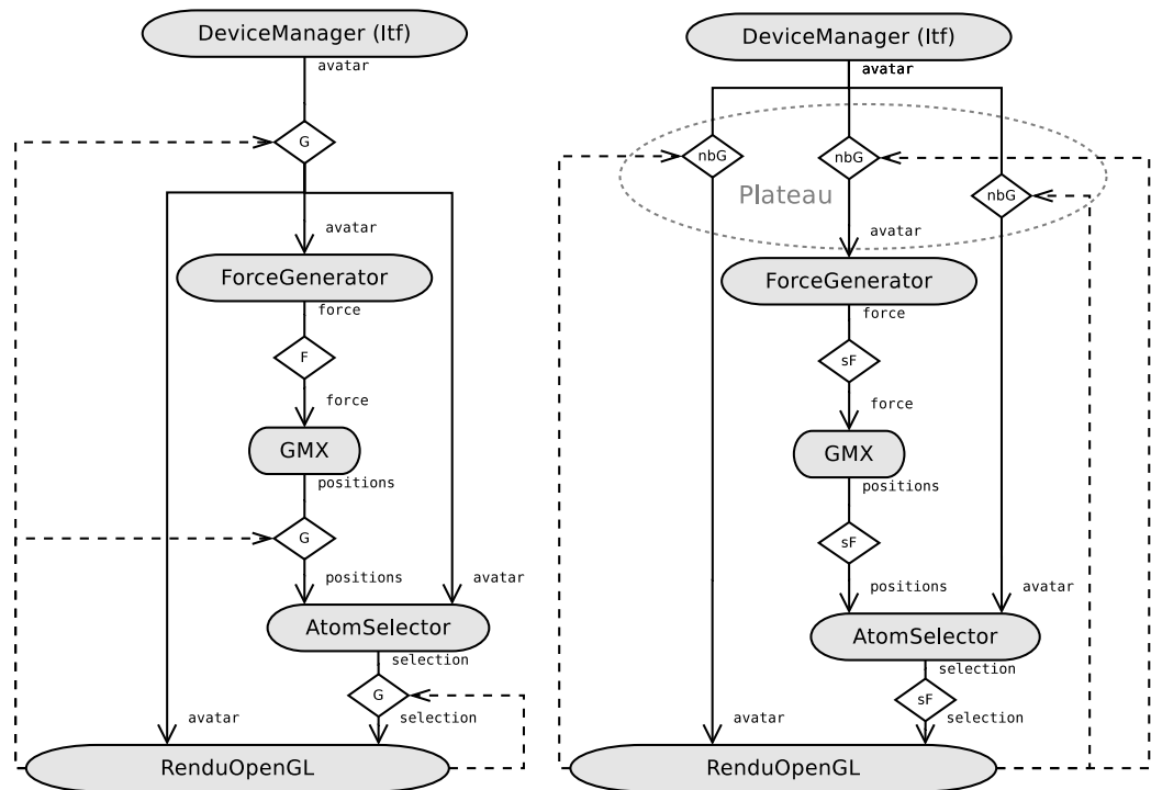
(a) Sous-graphe à partir de l'application manuellement construite
