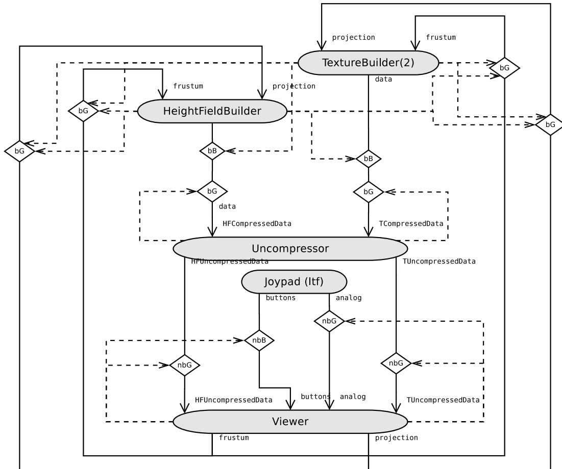
FIGURE 6.11 – Graphe d'application généré pour GeoCLOD.
