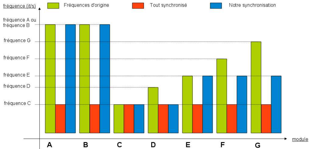
FIGURE 6.6 – Comparatif de performances entre trois types de synchronisation.
