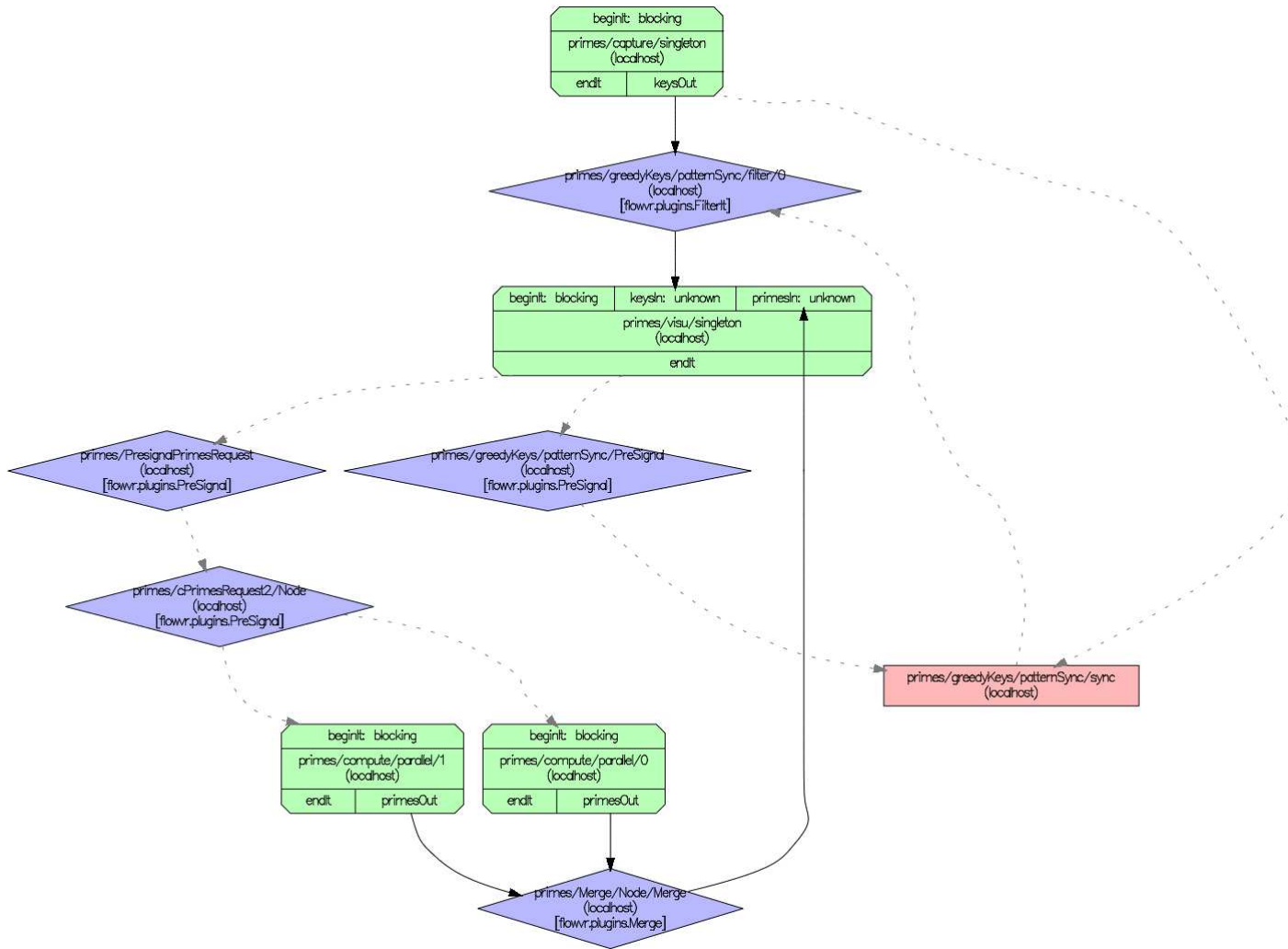
FIGURE 6.2 – Réseau FlowVR de l'application Primes où le module compute est parallélisé.
