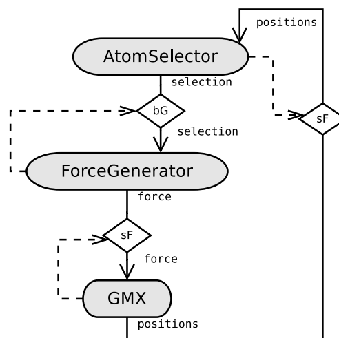
FIGURE 6.16 – Cycle synchrone initialement présent dans FVnano.
