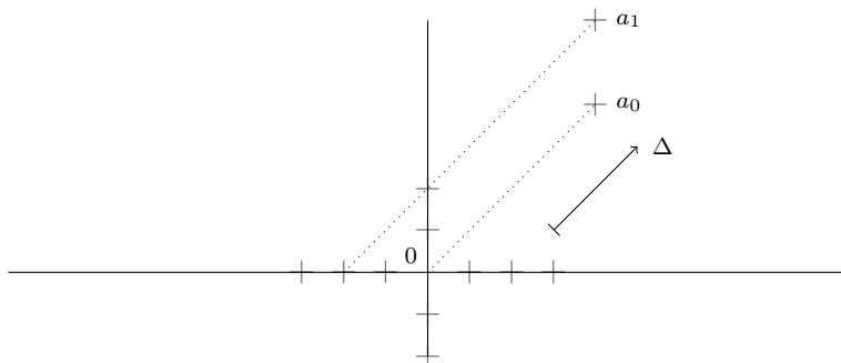
FIGURE 4 – a_0 et a_1 ont la même projection sur l'axe réel parallèlement à \exp\left(i\frac{\pi}{2}\right) , mais pas suivant \Delta qui est donc une direction admissible pour ces deux points.
