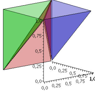
FIGURE 1 – Illustration du simplex D pour a = 0 et b = 1 .
