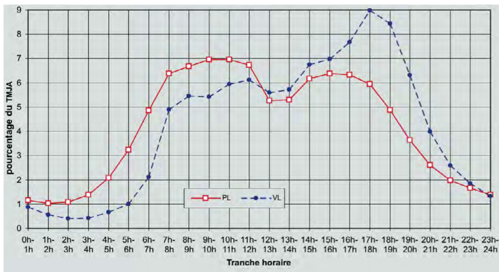
Figure 1.4 : profils moyens journaliers annuels de trafic Véhicules Légers (VL) et Poids Lourds (PL) sur Routes Nationales par tranche horaire. (source : Prédiction du bruit routier –
