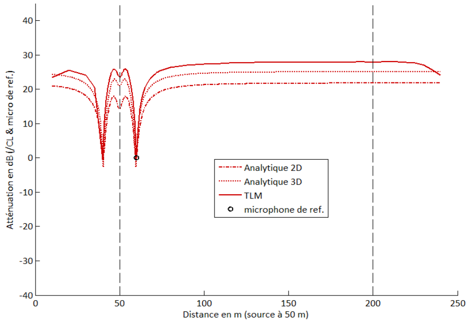
Figure 5.16 : validation de la TLM sur sol parfaitement réfléchissant.
