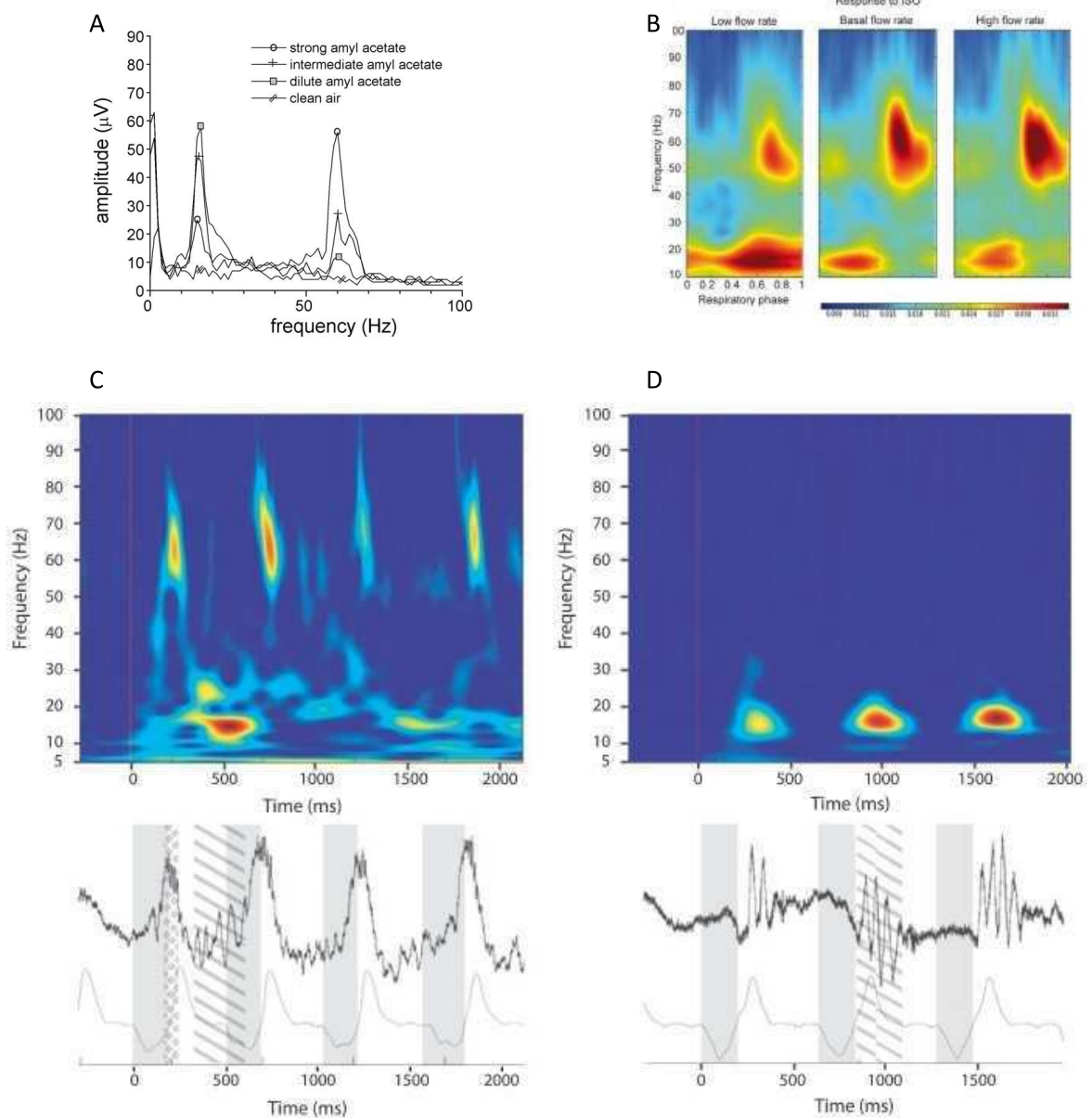
Figure I.10. Différentes réponses oscillatoires pour différents odorants chez le rat anesthésié. En haut : A. spectre des puissances pour différents types de stimulations : air pur ou concentration faible, intermédiaire et forte d'Acetate d'Isoamyl (Neville & Haberly, 2003). B. cartes temps/fréquence en réponse à l'acetate d'isoamyl avec un flux d'air variable : basal, faible et fort. A et B : dans les deux cas, les fréquences bêta sont favorisées par les faibles stimulations et les fréquences gamma par les fortes stimulations. C et D: En haut, cartes temps/fréquence représentant la puissance de l'oscillation (en code couleur) en fonction de la fréquence (en ordonnées) et du temps (en abscisses) avant et après l'odeur ( t=0 ) chez des animaux anesthésiés à l'urétrane. Bas : Signaux bruts et modulation respiratoire correspondants aux cartes temps/fréquence. C. Réponse à l'odeur d'éthyl pentanoate impliquant deux types d'oscillations : gamma en fin d'inspiration (losanges gris) avec un pic de puissance autour de 60 Hz, et bêta (hachuré) avec un pic de puissance autour de 15 Hz. D. Réponse à l'odeur d'hexanal induisant uniquement un pattern de réponse dans la bande bêta autour de 15 Hz. A noter : le bêta est légèrement décalé par rapport au cycle respiratoire comparé au profil mixte. Figure adaptée de Cenier et al., 2008.
