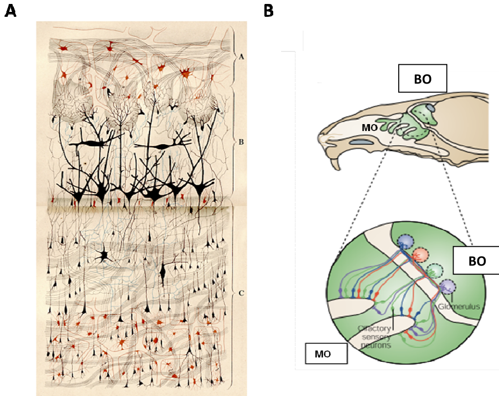
Figure I.1. Description anatomique du système olfactif. A. Planche dessinée représentant le bulbe olfactif principal (BO). Le marquage argentique permet de visualiser pour la première fois les circuits cellulaires du BO chez le rongeur (Golgi, 1875 ; figure modifiée de Shepherd et al. (2007)). B. Schéma d'une coupe sagittale d'une tête de rongeur. Le système olfactif est représenté en vert. Dans la cavité nasale se trouve la muqueuse olfactive (MO) qui contient les neurones olfactifs. Ces neurones traversent la lame criblée et atteignent le BO au niveau de structures sphériques appelées glomérules. Figure modifiée de Mombaerts (2004).
