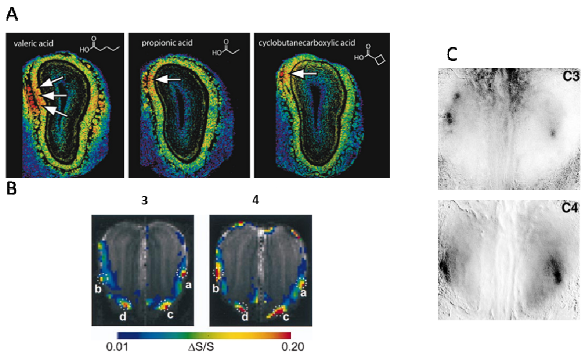
Figure I.4. Cartes d'activation spatiale du BO visualisées avec différentes techniques se basant sur des signaux endogènes liés au métabolisme énergétique. A. Cartes d'activation obtenues par imagerie 2DG en réponse à trois molécules portant des fonctions acides. Vue anatomofonctionnelle d'un hémibulbe (coupes coronales). B. Cartes d'activation (coupes coronales) obtenues par IRMf chez deux animaux différents (#3 et #4) en réponse à une exposition à l'isoamyl acetate 10^{-2} vapor pressure durant 4,8 minutes. Notons la reproductibilité des cartes chez les deux animaux. C. Cartes d'activation induites par du propanal (en haut) et butanal (en bas) obtenues par IOSI (vue dorsale). A. Figure modifiée de Johnson & Leon., 2007. B. Modifiée de Yang et al., 1998. C. Modifiée de Belluscio & Katz., 2001.
