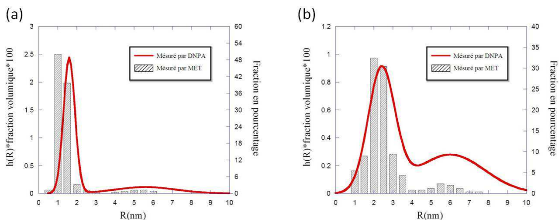
Figure 3-9 : Comparaison des histogrammes de tailles des nanoparticules déduits des observations directes en MET et des mesures de DNPA sur (a) : l'échantillon B et (b) : l'échantillon C.
