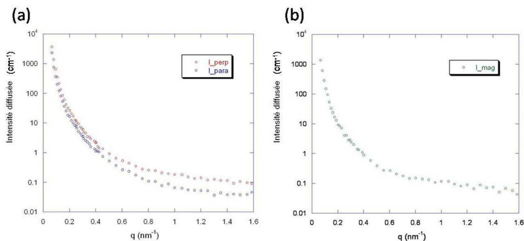
Figure 3-1 : Intensité diffusée (a) perpendiculairement et parallèlement au champ magnétique, et (b) intensité magnétique diffusée en fonction de q, mesurées sur la poudre co-broyée du matériau de référence.
