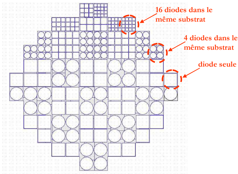
Fig.II.1. – Layout du masque des diodes de puissance avec terminaisons en tension verticale.
