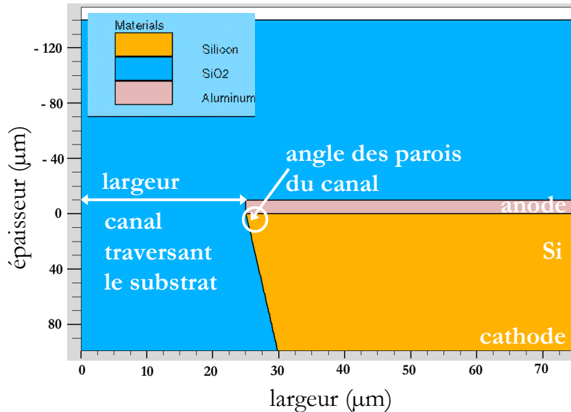
Fig. III.38. – Vue en coupe de la structure de la diode de puissance avec DRIM Cooler.
