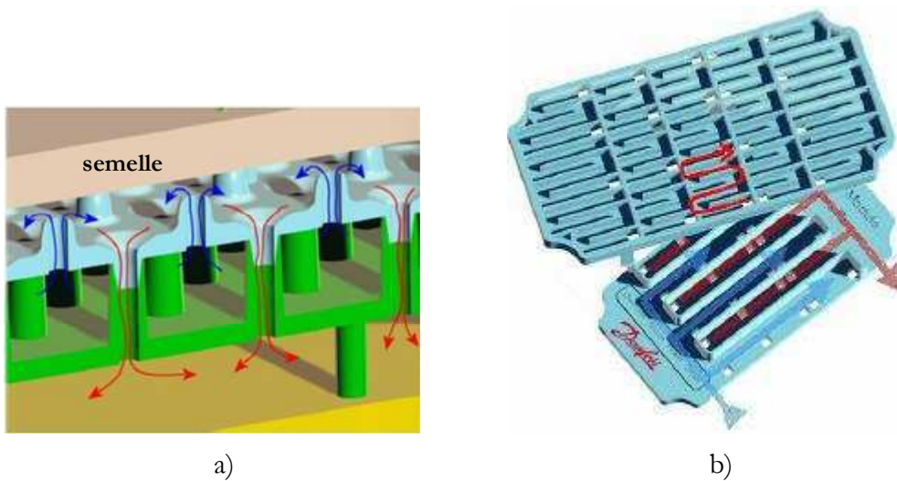
Fig. I.28. - Concept Shower Power a) jets impactant la semelle du module et b) canaux sinusoïdaux [OLE06].
