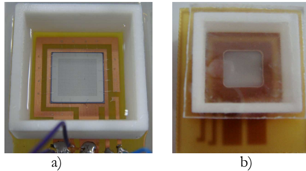
Fig.II.20.- Photos du package des diodes avec DRIM Cooler passivées avec de l'huile silicone a) face avant et b) face arrière.
