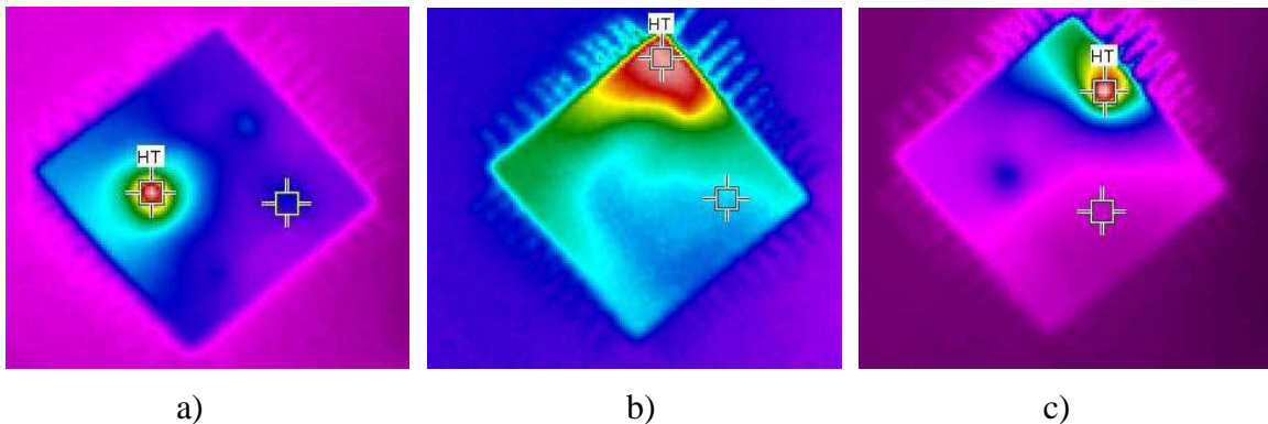
Fig. IV.21. – Mesures avec une camera infrarouge de la température en surface d'une diode avec DRIM Cooler a) T_{\text{max}} = 84.4^{\circ}\text{C} et T_{\text{min}} = 41.3^{\circ}\text{C} , b) T_{\text{max}} = 51.7^{\circ}\text{C} et T_{\text{min}} = 35^{\circ}\text{C} et c) T_{\text{max}} = 215^{\circ}\text{C} et T_{\text{min}} = 44.2^{\circ}\text{C} .
