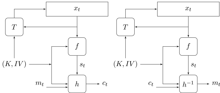
FIGURE 1.2 – Chiffrement à flot synchrone et déchiffrement associé
