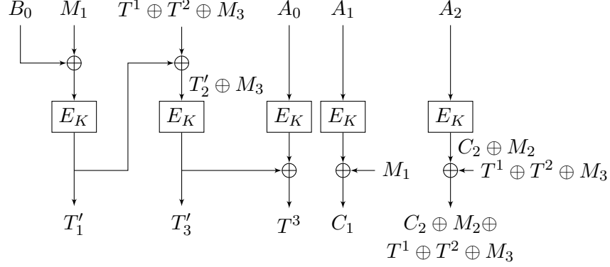
FIGURE 4.5 – Attaque de CCM sans tenir compte de la taille des données
