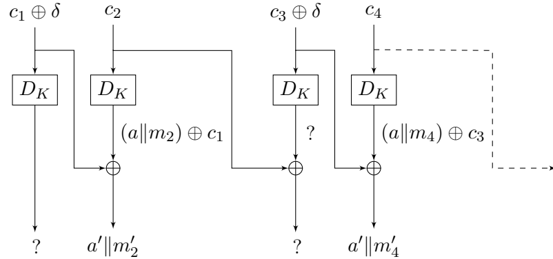
FIGURE 4.13 – Une (autre) attaque contre CBC-AREA
