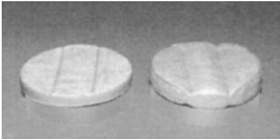
(a) (b) Figura 3.8 – Amostras de GCL costurado hidratados (a) com sobrecarga (b) sem sobrecarga (Vangpaisal & Bouazza, 2004).
