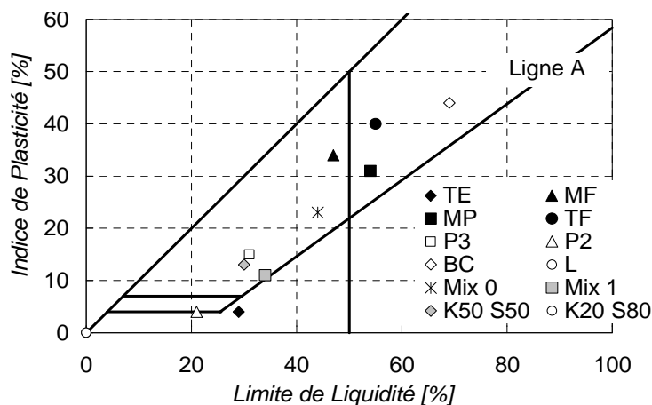
Figure III-1: Position des différents sols sur le diagramme de Casagrande.
