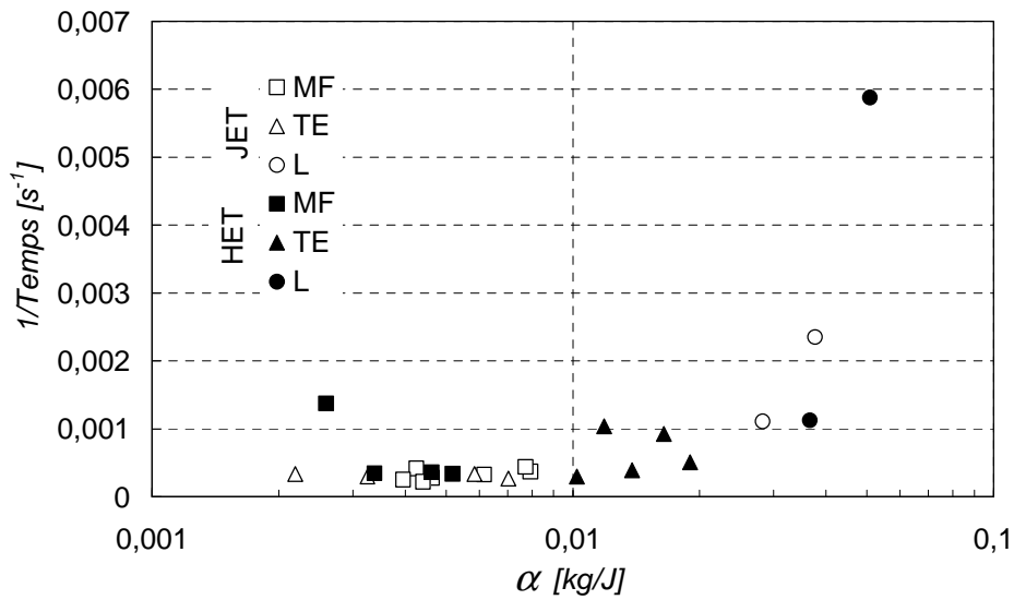
Figure III-23 : Diagramme inverse du temps d'érosion en fonction de alpha, petite échelle de variation.
