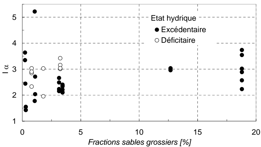
Figure 7 : Indice d'érodibilité en fonction de la fraction de sable > 425 \mu m .
