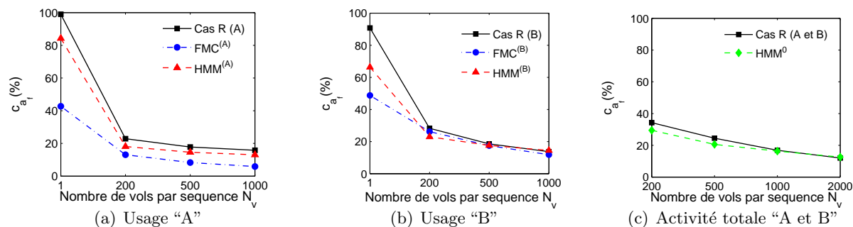
Figure 4.5 – Coefficient de variation c_{a_f} de la profondeur de fissure a_f (pour N_T = 6000 vols) en fonction du nombre de vols par séquence N_v et du mode de simulation choisi (cas R, cas S : FMC ou HMM).
