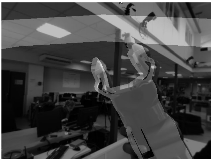
FIGURE 4.15 – Reprojection du modèle du robot dans l'image captée par une caméra embarquée pour valider la calibration des paramètres de cette dernière.
