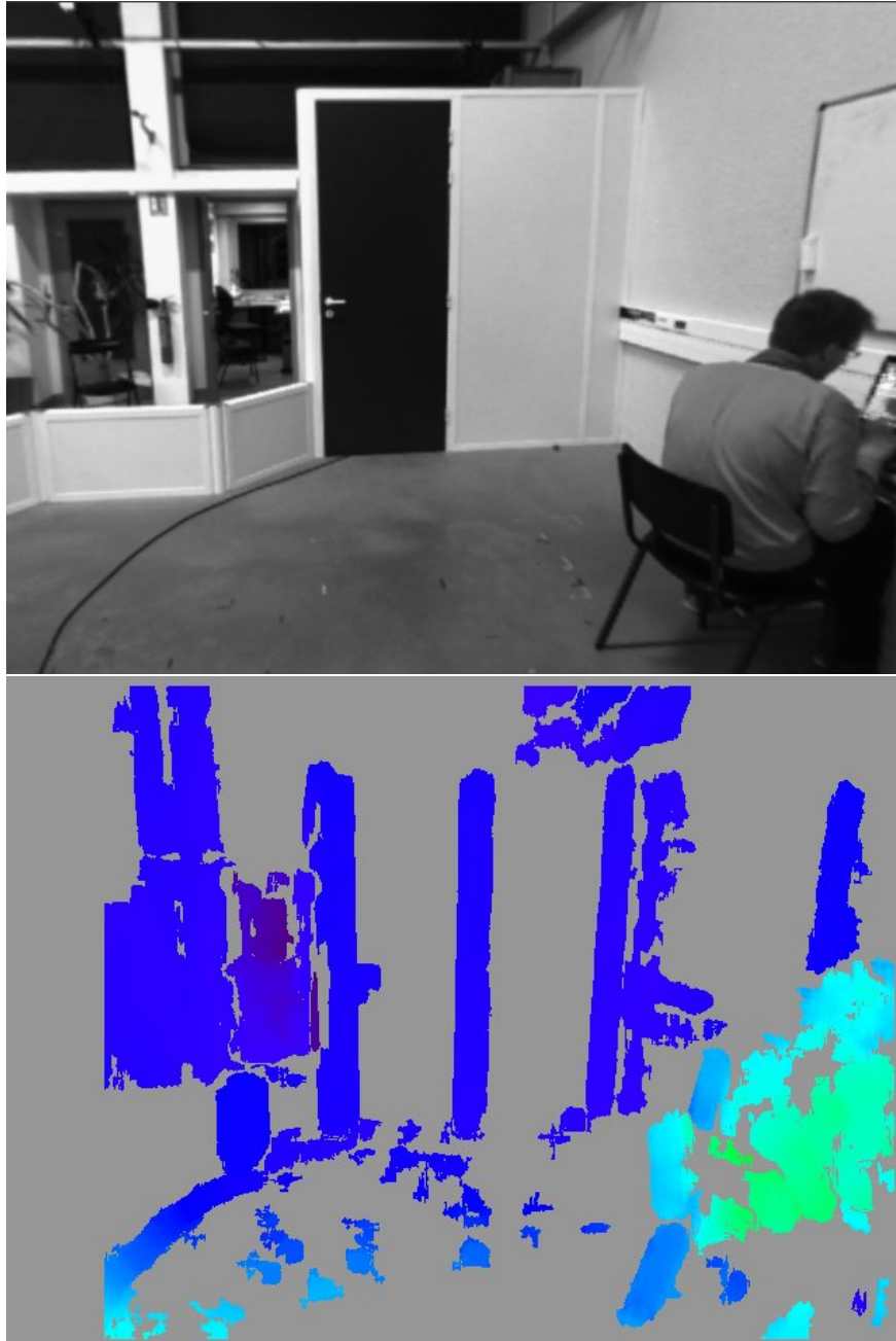
FIGURE 5.3 – Carte de profondeur calculée en temps réel. Une couleur claire correspond à une faible profondeur, une couleur foncée à une profondeur importante. Les zones grises indiquent les endroits où aucune correspondance n'a pu être établie entre les images de deux caméras. Elles correspondent typiquement à une zone peu texturée comme un mur.
