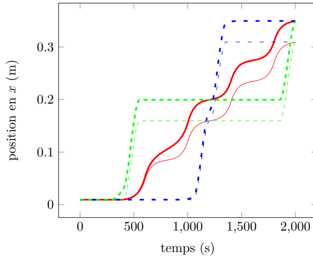
FIGURE 3.5 – Évolution, pendant deux pas, de la position en x du centre de masse (—), du pied gauche (- -) et du pied droit (- - -). La courbe en gras illustre un pas de 0.3m en avant. Les courbes en pointillé illustre la position du centre de masse (—), pied gauche (- -) et pied droit (- - -) après un pas de 0.05m en avant, soit une correction de 0.02m.
