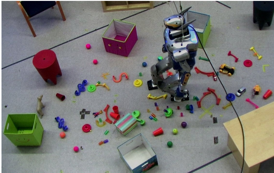
FIGURE 3.7 – HRP-2 marchant dans un environnement extrêmement encombré tout en évitant des obstacles. La position finale est atteinte avec une précision de \pm 3\text{cm} . L'erreur finale est la conséquence du bruit impactant l'estimation de la position du robot ainsi que de la dérive accumulée sur la fin de la trajectoire qu'il n'est pas possible de corriger, faute de temps.
