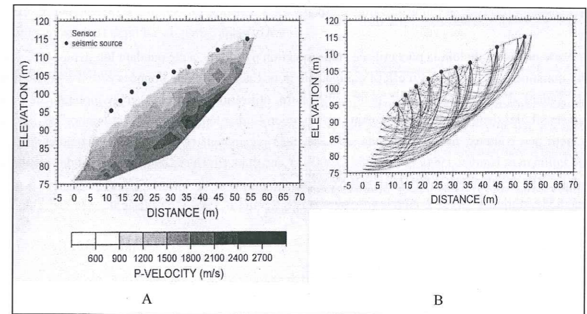
Figure IV.A-3 Exemple de panneau de tomographie sismique (A) et trajets des rais associés (B) sur le glissement de terrain de Bas-Oha, Belgique (Jongmans et al., 2000)
