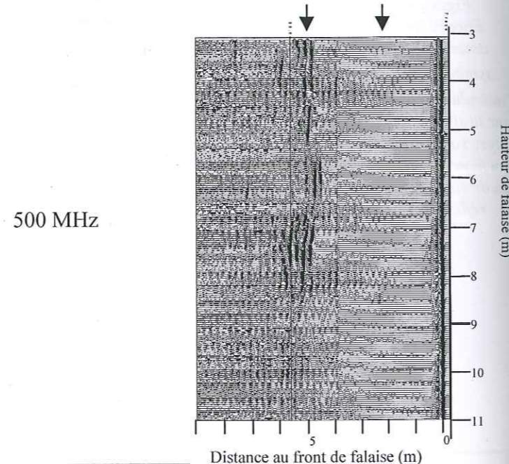
Figure IV.C.15. Profil P'.3 : Enregistrements radar avec les antennes 120 et 500 MHz. Les flèches indiquent les réflecteurs qui correspondent à des discontinuités observées sur le terrain. Ces discontinuités sont schématisées dans l'encadré, avec leur position mesurée par rapport au front de falaise, orthogonalement à leur direction.
