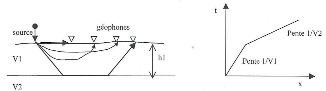
Figure IV.A-1. Schéma de principe d'un profil de sismique réfraction et son hodochrone associée dans le cas idéal d'un bicouche horizontale
