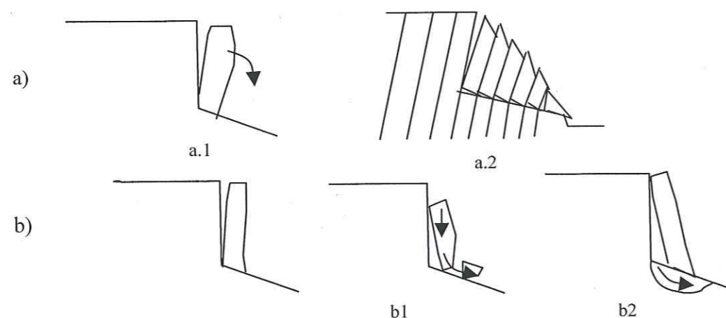
Figure III.B-8. Exemple de mécanismes possibles de rupture de colonne: a) Basculement de colonnes ou de blocs ; b) Rupture de colonne en pied.
