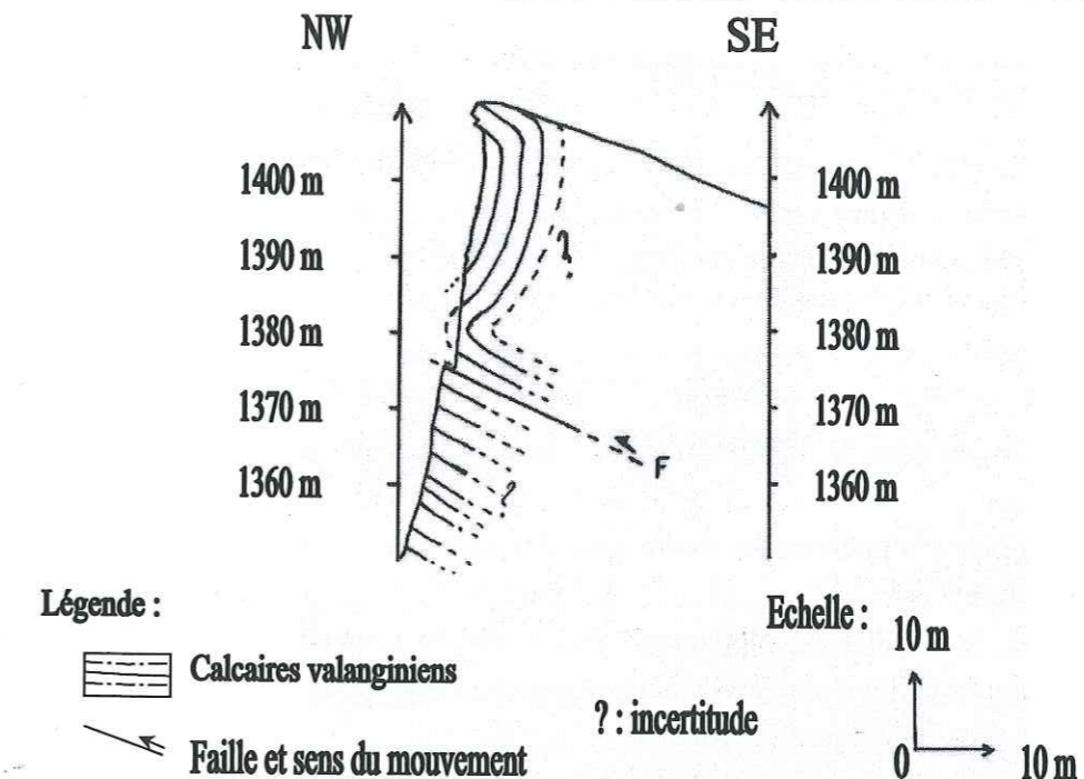
Figure II.B-13. Coupe géologique interprétative de la falaise du Pas de l'âne au niveau de l'éboulement de 22/03/96 (d'après Taluy, 2000).
