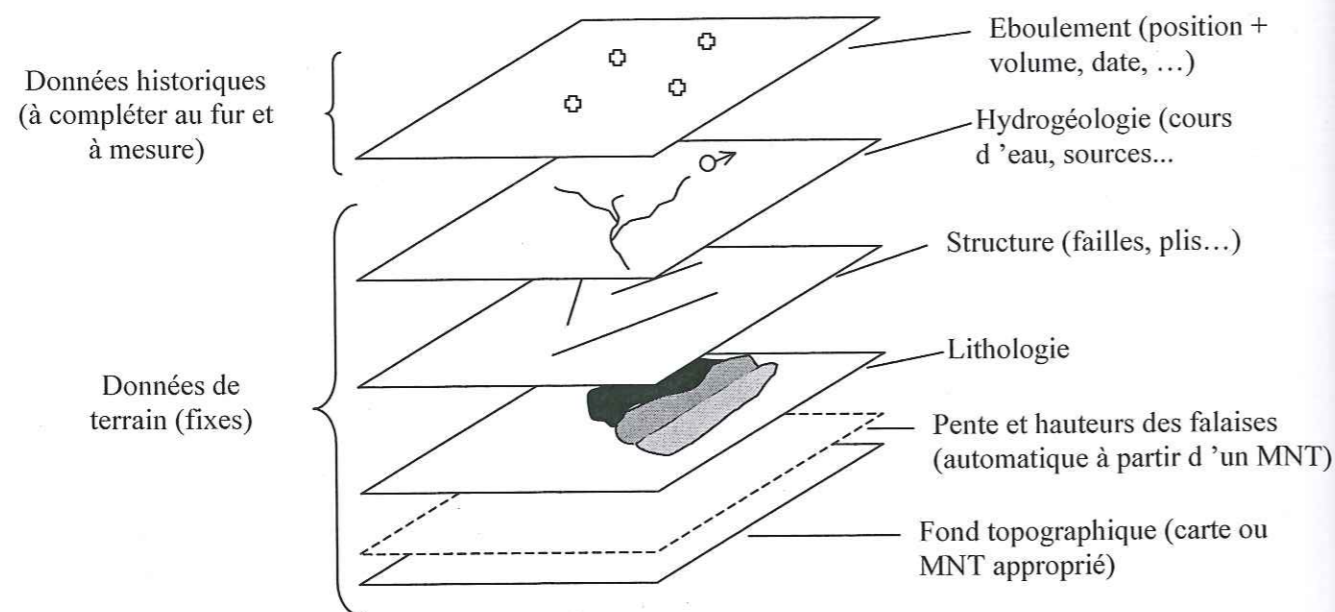
Figure II.D-1. Principe de superposition des couches d'information dans un Système d'Information Géographique
