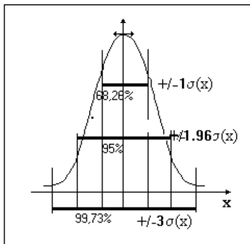
fig n°C 11 estimation en pourcentage pour des valeurs spécifiques
