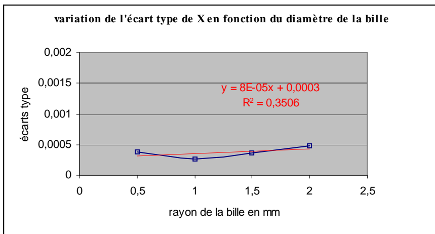
graphique n°3 28 Variation de l'écart type de x en fonction du diamètre de la bille
