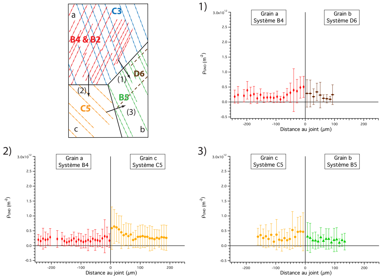
FIGURE II.25 – Évolution de la densité de dislocations moyenne, mesurée à partir de l'étalement des pics dans la direction théorique d'étalement pour chaque système activé, avec la distance au joint. Les barres d'erreurs correspondent à l'écart-type sur les valeurs moyennées.
