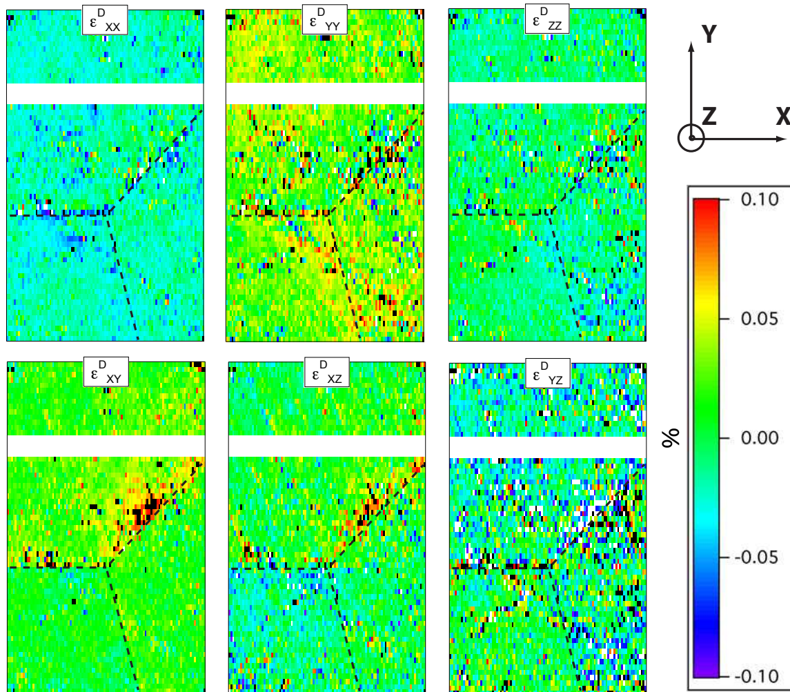
FIGURE II.30 – Évolution des six composantes du tenseur déviateur des déformations élastiques locales induites par la déformation de l'échantillon.
