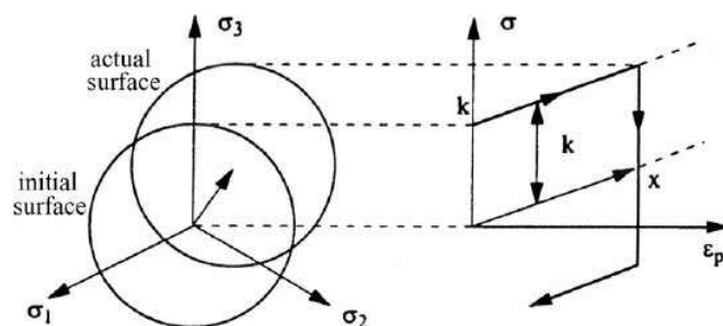
FIGURE I.26 – Principe de l’écrouissage cinématique : l’écrouissage se traduit par un déplacement de la surface de charge dans une direction donnée. Un premier chargement suivi d’une décharge entraîne notamment un abaissement de la limite élastique dans la direction de sollicitation inverse à celle du premier chargement (effet Bauschinger). (D’après Chaboche (2008))
