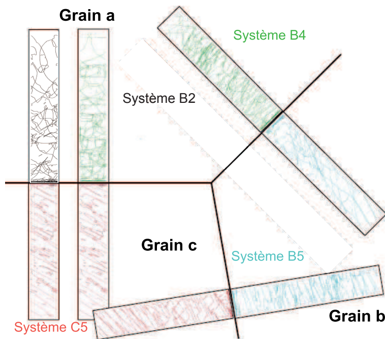
FIGURE III.4 – Schéma illustrant la reproduction des configurations d'orientation joint de grains - systèmes de glissement activés sur le tricristal expérimental, par le biais de simulation de DD plastique - plastique.
