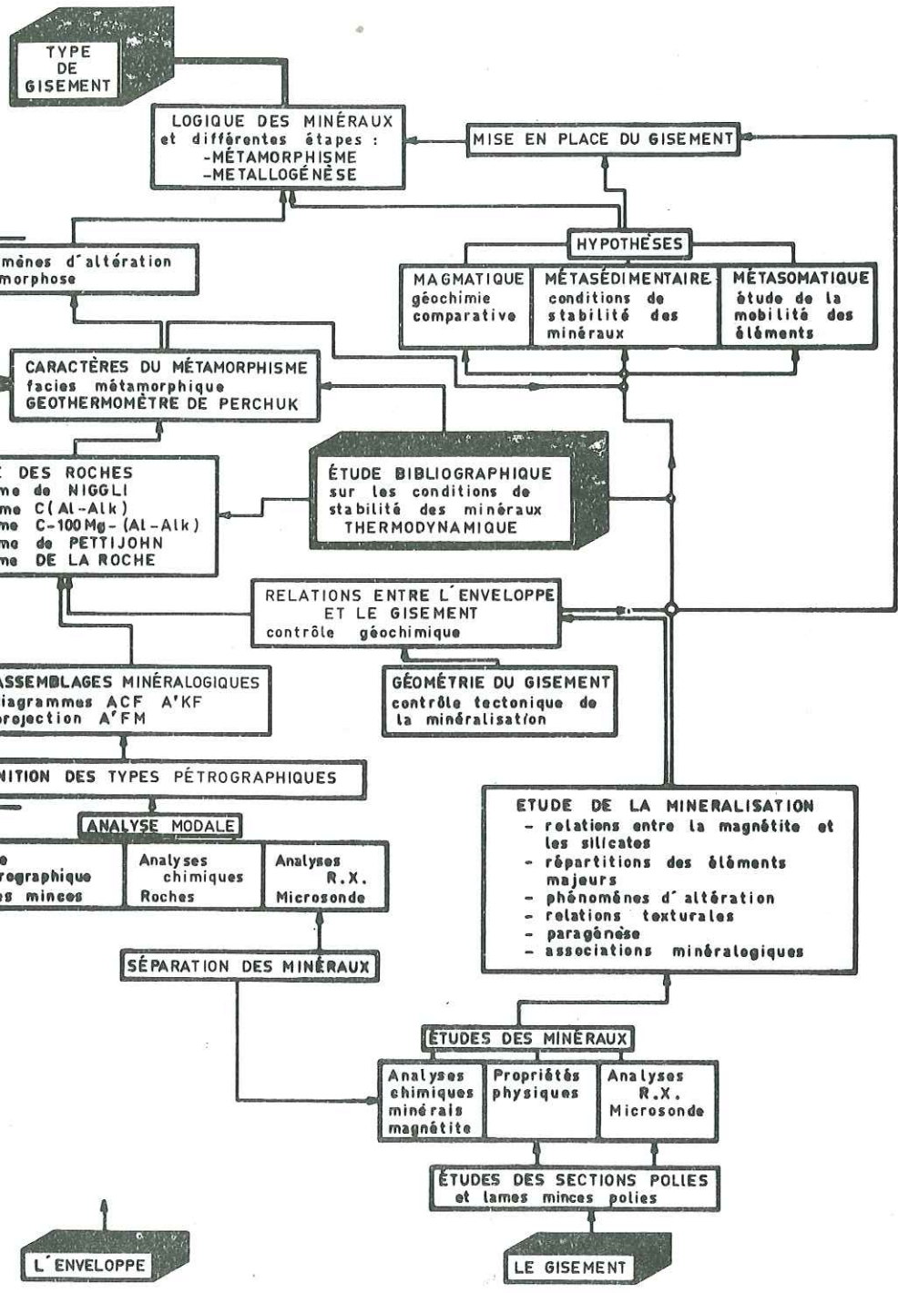
SCHEMA METHODOLOGIQUE DE L'ETUDE DU GISEMENT DE MAGNETITE DE HULL IRON
