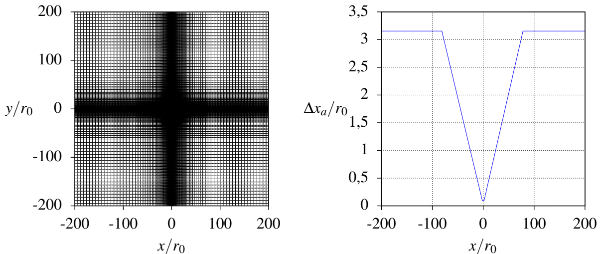
FIG. 5.5: Maillage acoustique.
