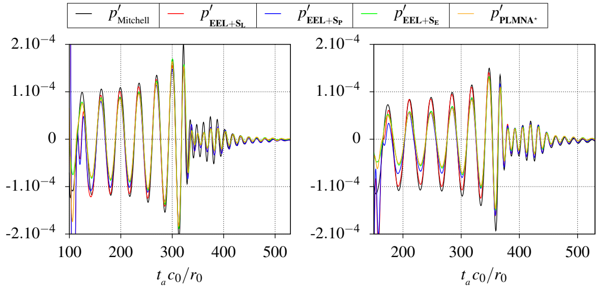
FIG. 5.37: Comparaison de l'évolution temporelle de p' obtenue par les diverses formulations au point A à gauche et au point B à droite.
