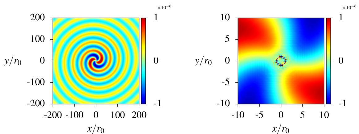
FIG. 5.15: Pression acoustique   t_a c_0 / r_0 = 1000 calcul e dans la configuration ck1 avec PLMNA* . Zoom sur la partie centrale   droite .
