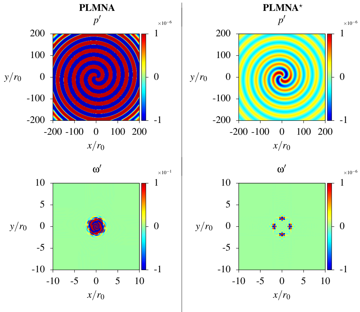
FIG. 5.14: Solutions à t_a c_0 / r_0 = 500 calculées dans la configuration ck1 avec PLMNA à gauche, PLMNA* à droite. En haut, pression acoustique p' ; en bas, vorticit  perturb e \omega' .
