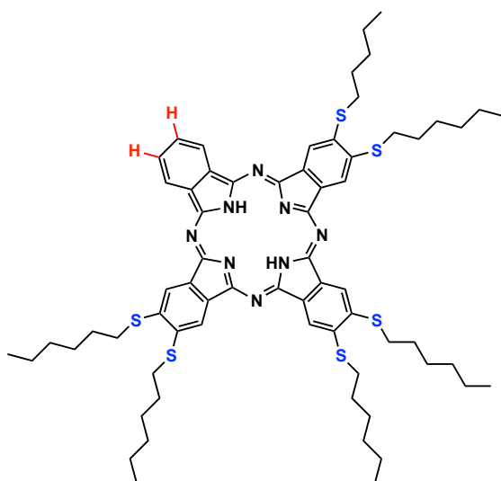
AB3 (6)
