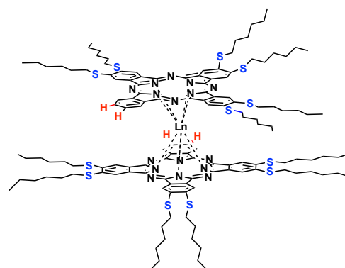
Ln(AB3) 2
