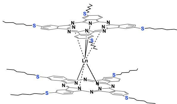
Ln(T4) 2
