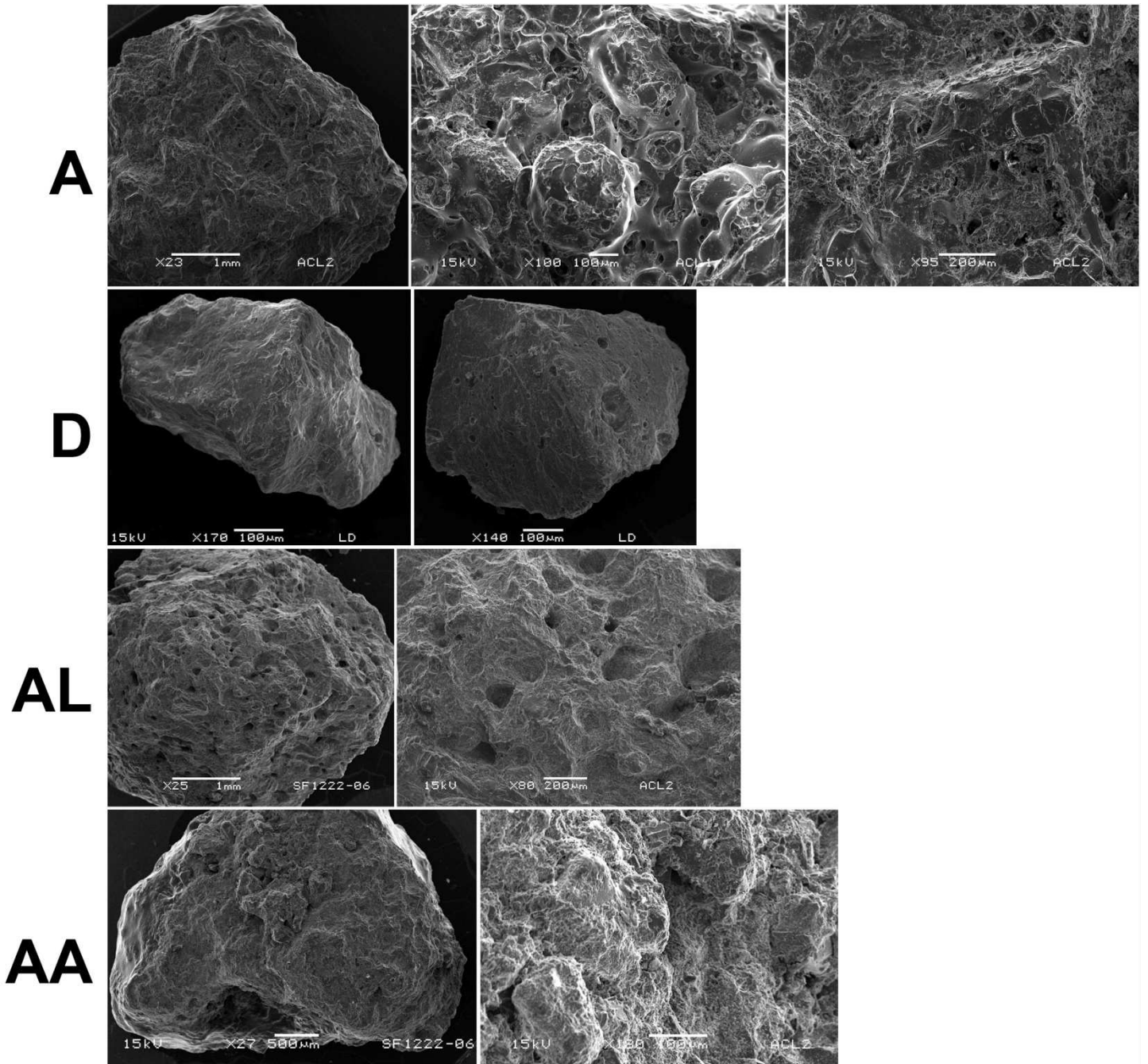
Figure 5.6 : Images de particules et de détails de surface de grains issus des classes de constituants (A) agrégats de cristaux, (D) lithiques denses, (AL) lithiques altérés et (AA) agrégats de cendres. Images MEB en électrons secondaires.
