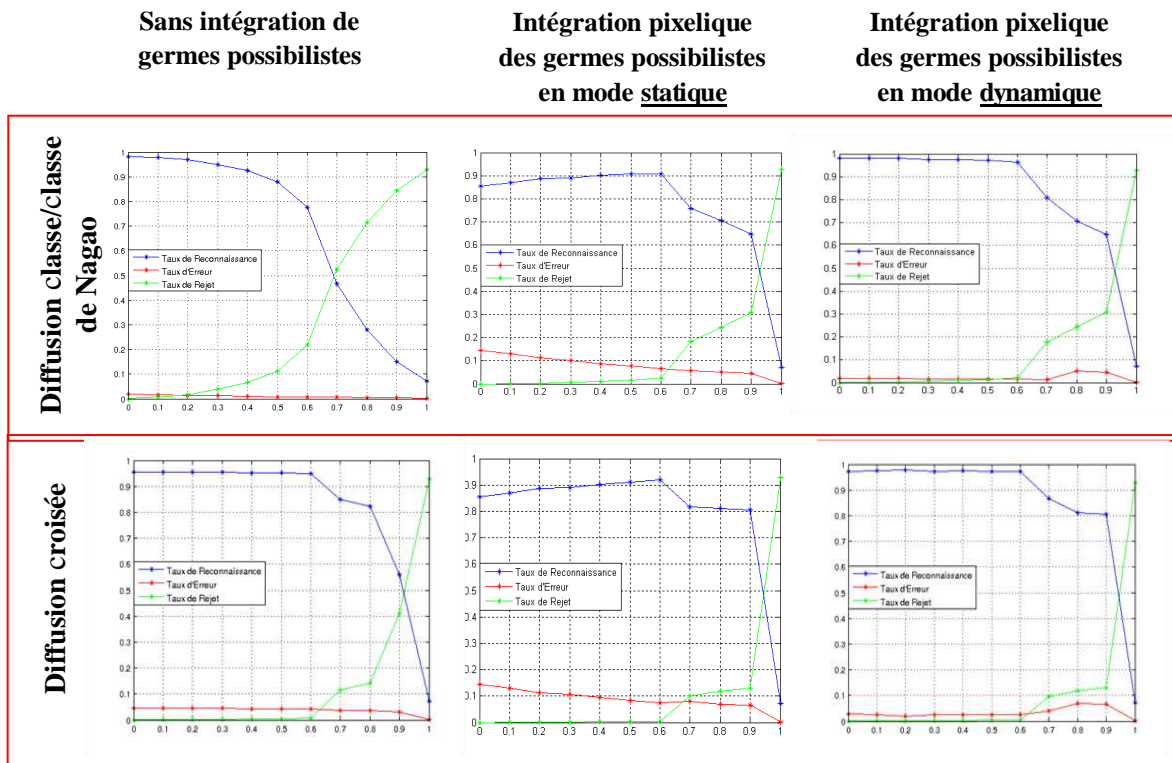
Figure 5.8 : Taux de reconnaissance, d'erreur et de rejet (en fonction du seuil) sans intégration et avec intégration pixelique (en modes statique et dynamique) des germes possibilistes au processus de propagation des connaissances, par diffusion classe/classe de Nagao et diffusion croisée
