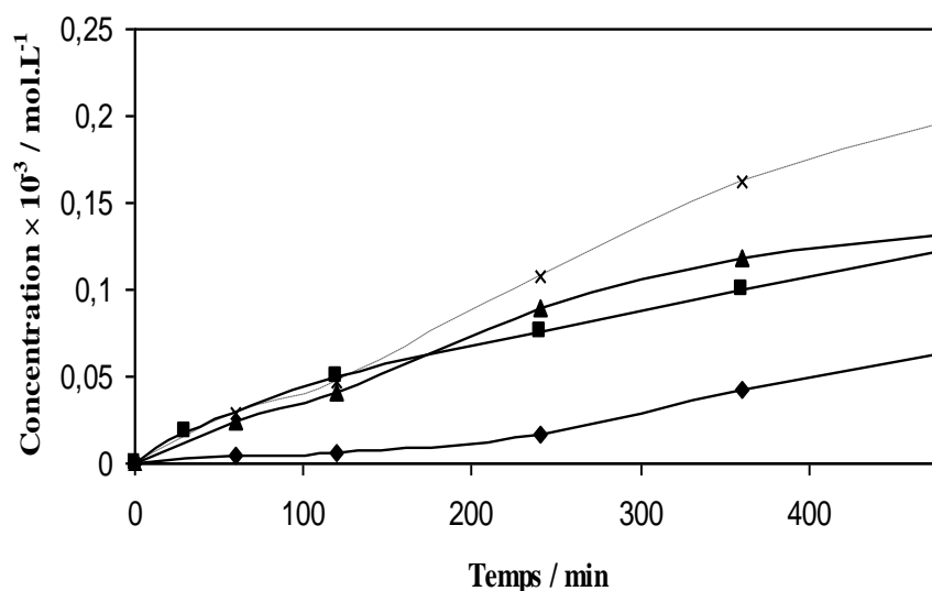
Figure IV-16. Évolution des ions nitrate, ammonium et sulfate au cours de l'électrolyse du bentazone. [\text{Bentazone}]_0 = 0,125 \times 10^{-3} \text{ mol L}^{-1} , [\text{Fe}^{3+}] = 0,1 \times 10^{-3} \text{ mol L}^{-1} (catalyseur), I = 100 \text{ mA} . (◆) nitrate, (■) sulfate, (▲) ammonium, (×) azote totale.
