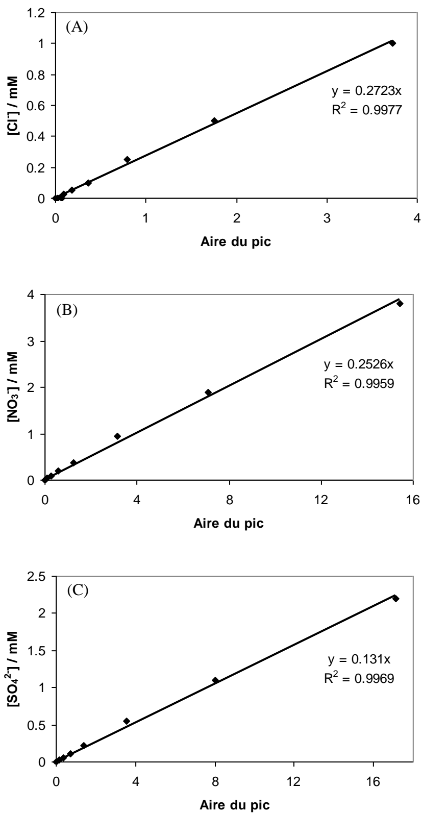
Figure II-6. Courbes de calibration obtenues pour le dosage des anions : (A) \text{Cl}^- , (B) \text{NO}_3^- et (C) \text{SO}_4^{2-} .
