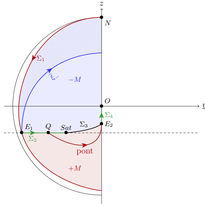
FIGURE 3.2 – Synthèse optimale partant du pôle nord, pour un seul spin : les \Sigma_i forment le lieu de commutation séparant les régions +M et -M respectivement en rouge et bleu. L'arc bang \bar{\xi}_- sépare les deux domaines, l'un bang-bang (hachuré) et l'autre avec un arc singulier non trivial. La trajectoire optimale pour rejoindre le centre en temps minimal est NE_1QE_2O . Le reste de la synthèse s'obtient par symétrie.
