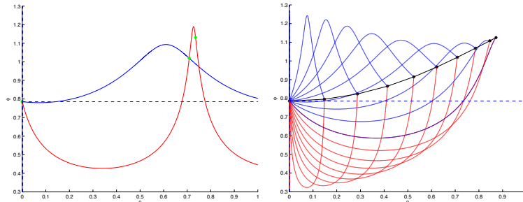
FIGURE 4.4 – Des extrémales petites s'intersectant pour différents niveaux du Hamiltonien avec le même coût, p_r = 0 , \delta = 4 , \varphi_0 = \pi/4 . À gauche, la première intersection arrive en t_f = 1 pour h \simeq -1.095 (bleu) et h \simeq -9.486e^{-1} (rouge), respectivement. À droite, une famille entière de telles paires s'intersectant en t_f = 1 avec le même coût est affichée. Ces intersections génèrent la partie II du lieu de coupure, voir Figs. 4.5-4.9.
