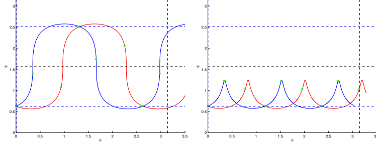
FIGURE 4.3 – Des extrémales s'intersectant, avec la symétrie \pm\dot{\varphi}(0) . Une paire d'extrémales grandes ( \xi^2 > 0 ) sur la gauche, une paire de petites ( \xi^2 < 0 ) sur la droite, chacune s'intersectant avec le même coût pour t_f égal à la période de X = \sin^2 \varphi . Dans chacun des cas, les extrémales s'intersectant appartiennent au même niveau du Hamiltonien. Ces intersections génèrent des points de coupure I.a (pour les grandes) et I.b (pour les petites), voir Figs. 4.5-4.9. Ces points appartiennent respectivement à la ligne antipodale \varphi = \pi - \varphi_0 et à \varphi = \varphi_0 .
