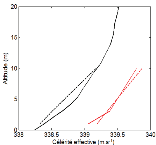
Figure 7.19 : profils moyens (mâts à 50 et 150m de la source) de célérité effective selon DP3 pour le cas NEUT issus de Meso-NH (noir) et de l'expérience (rouge) et de leurs profils linéaires estimés à partir du gradient (traits pointillés).
