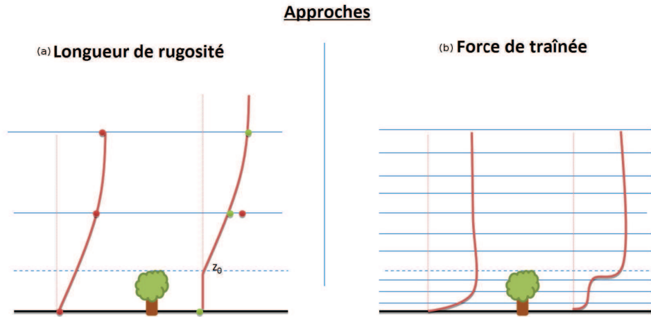
Figure 4.7 : schéma représentant le profil de vent typique en présence de végétation modélisé par la longueur de rugosité z_o (a), puis par le modèle en force de traînée (b).
