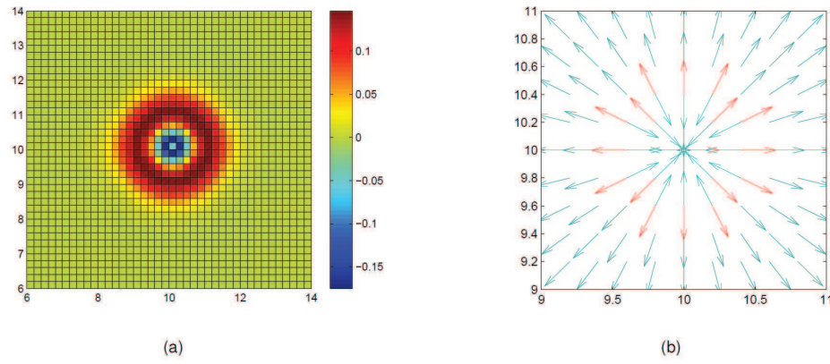
Figure 5.23 : tracé de l'amplitude d'une onde (a) et de son intensité (b). La direction théorique du front d'onde (en rouge) peut se trouver opposée à la direction du vecteur intensité (en bleu).
