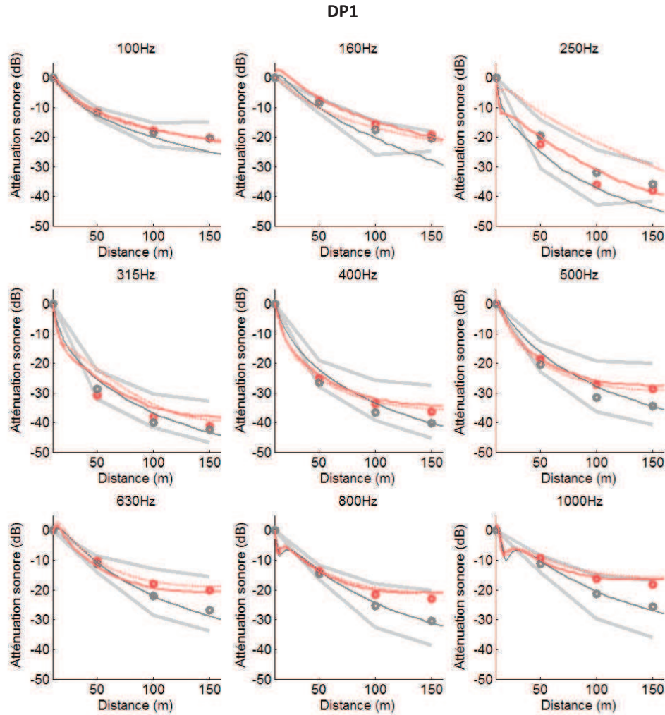
Figure 7.7 : niveaux sonores mesurés (cercles) et simulés (TLM : trait plein, EP : trait pointillé) pour le cas NEUT - profil linéaire (rouge) et en conditions homogènes (gris) pour DP1. ( \sigma = 150 cgs, la dispersion expérimentale des niveaux sonores sur toute la campagne est encadrée par les traits gris clairs).
