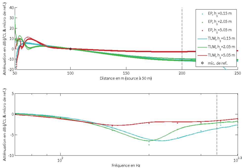
Figure 5.24 : validation de la TLM sur sol absorbant en présence d'un gradient vertical de vent. Atténuation sonore du signal par rapport au champ libre (CL) et par rapport à un microphone de référence à 50 m de la source ( dist_{obs}=150 \text{ m} ) et de la fréquence ( f_{obs}=200\text{Hz} ).
