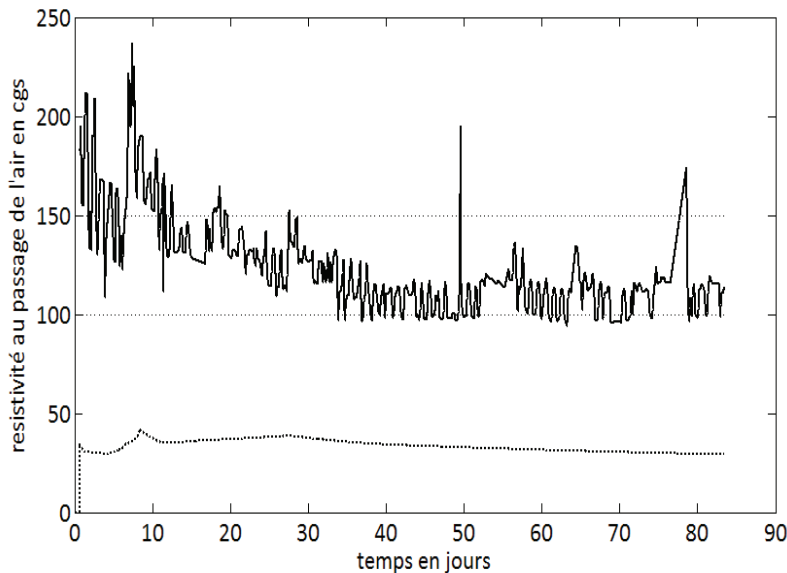
Figure 3.2 : mesures de la résistance au passage de l'air du sol \sigma lors des 3 mois de mesures de la campagne expérimentale de Lannemezan 2005. Moyenne (-) et écart type (...) sur tous les capteurs présents sur la zone.
