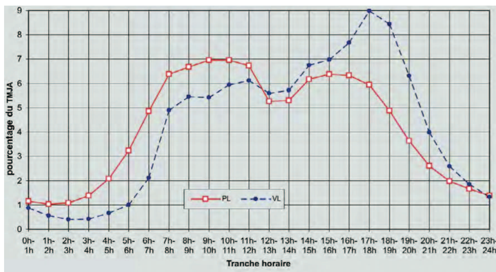
Figure 1.4 : profils moyens journaliers annuels de trafic Véhicules Légers (VL) et Poids Lourds (PL) sur Routes Nationales par tranche horaire. (source : Prévission du bruit routier – SETRA [7])
