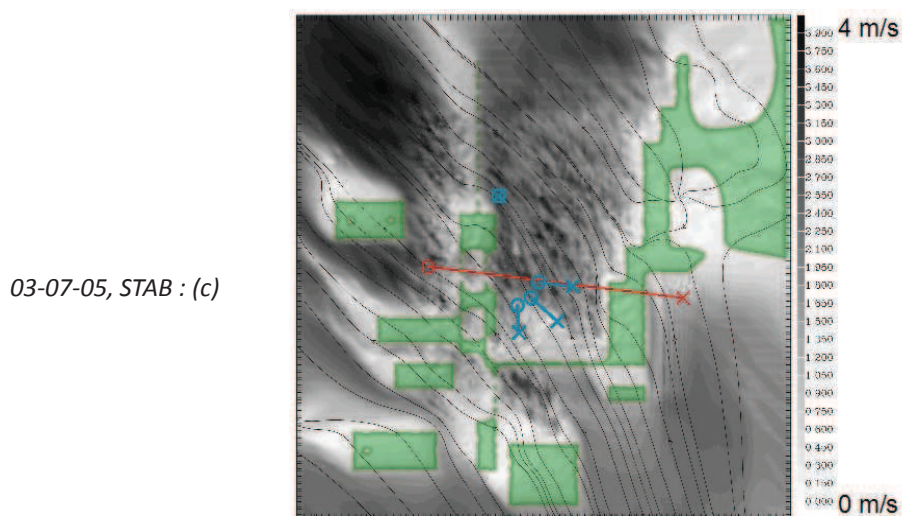
Figure 6.1 : coupe horizontale du champ de vent instantané à 10 m du sol sur la zone expérimentale de Lannemezan 2005. En bleu, le positionnement des capteurs de mesures, les zones vertes correspondent aux zones arborés. (a : 16/06/05, b : 17/06/05, c : 03/07/05)
