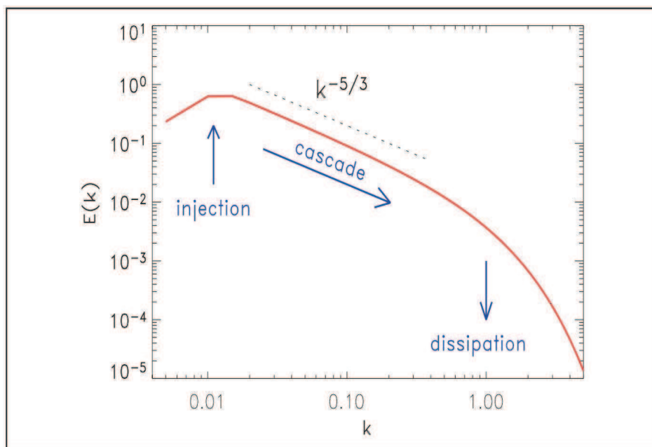
Figure 2.6 : représentation schématique du spectre de Kolmogorov.
