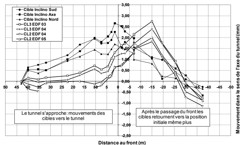
Figure 5.14 Mouvements des cibles analysés selon la direction de l'axe du tunnel
