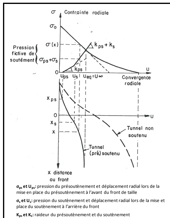
Figure 1.11 Méthode convergence-confinement avec prise en compte du présoutènement (Guilloux et al. [1996])
