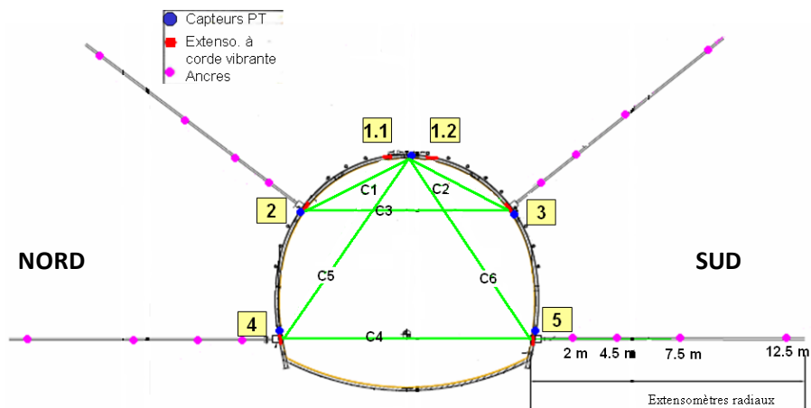
Figure 6.11 Mesures et instruments en souterrain
